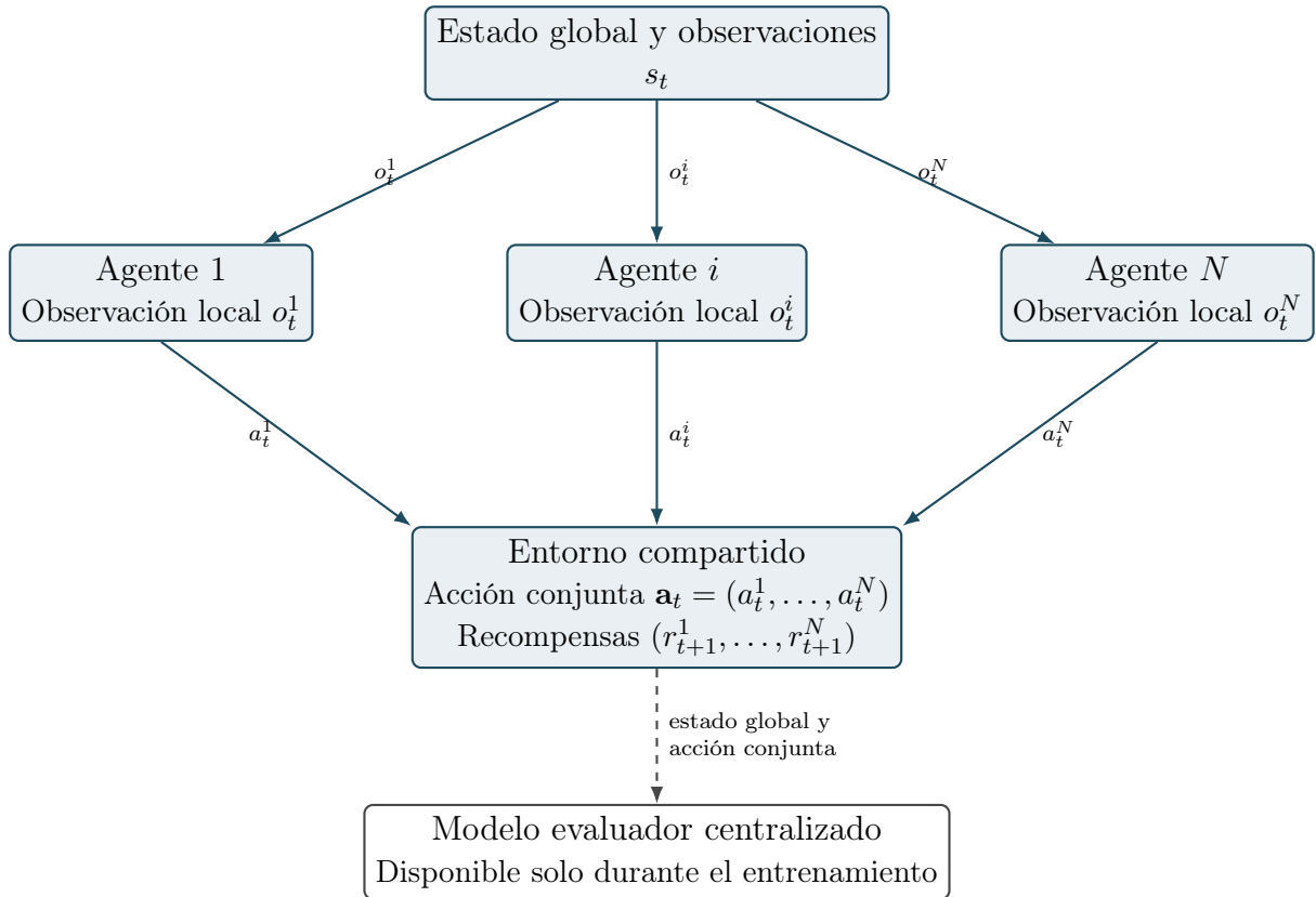
Figura 2.2: MARL con entrenamiento centralizado y ejecución descentralizada.
