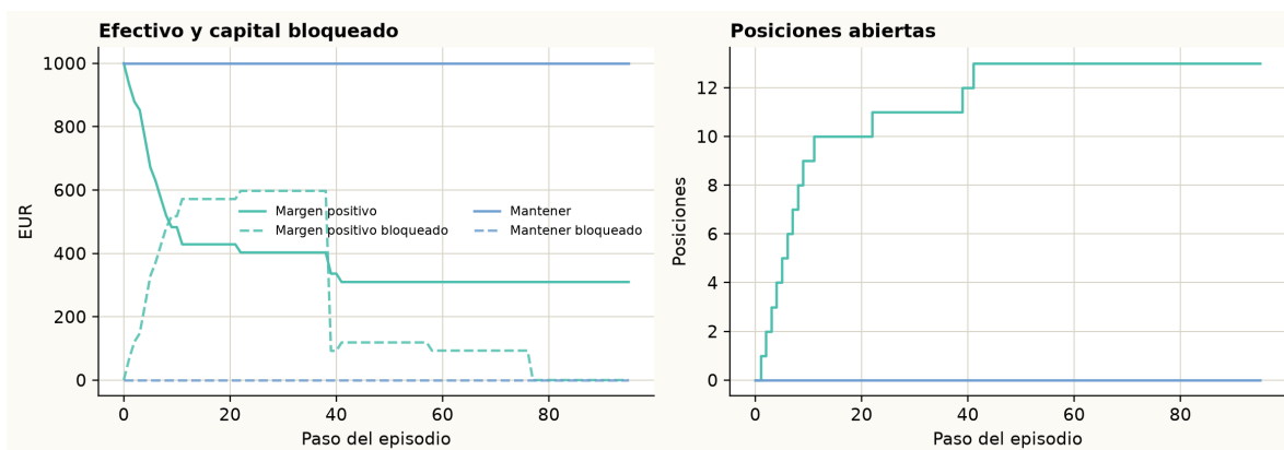
Figura 7.6: Trazas MARL.
