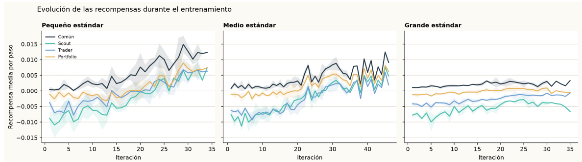
Figura 7.5: Recompensas durante el entrenamiento.
