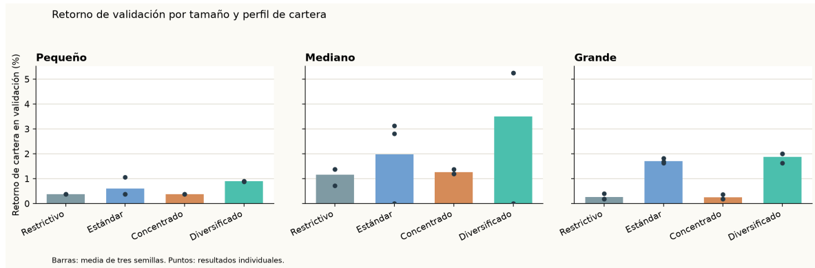
Figura 7.8: Retorno de validación por escenario.
