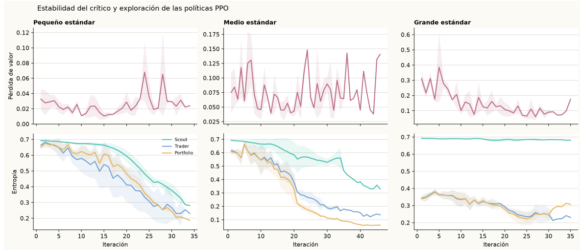
Figura 7.6: Estabilidad del entrenamiento con PPO.
