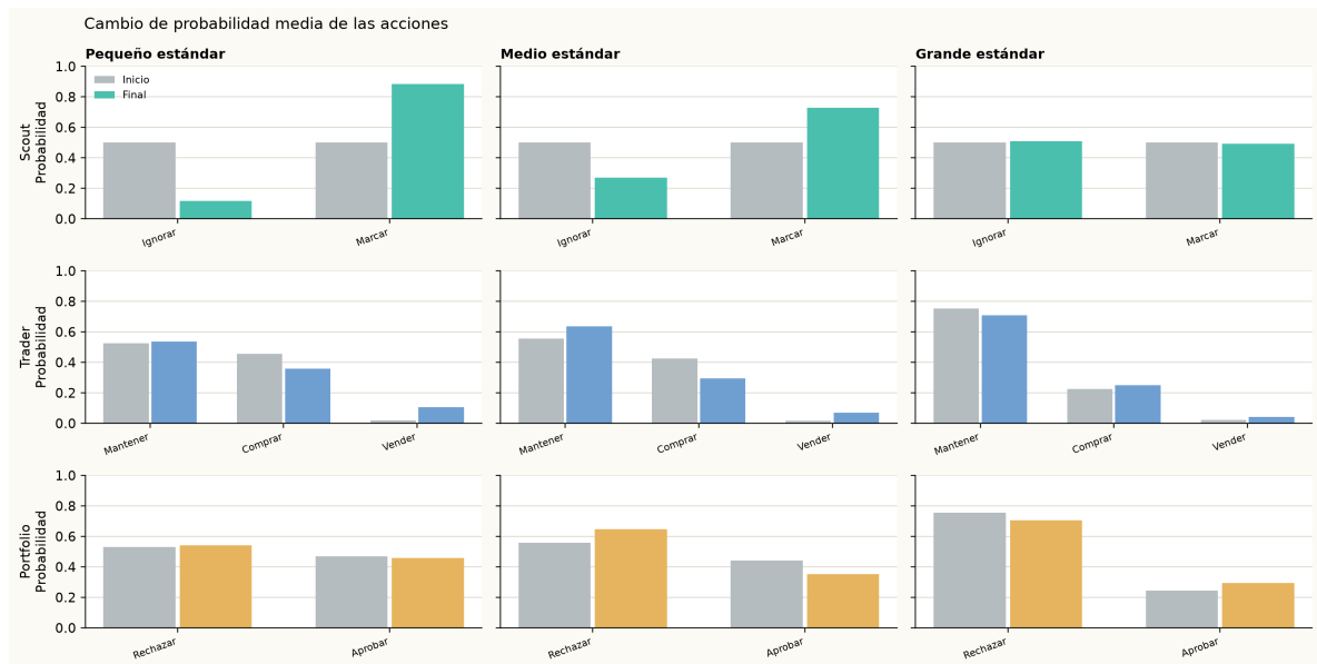
Figura 7.7: Políticas al inicio y al final del entrenamiento.
