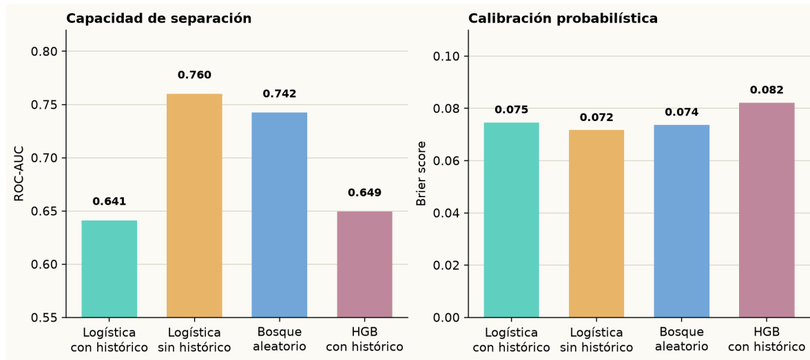
Figura 7.2: Modelos en marzo.
