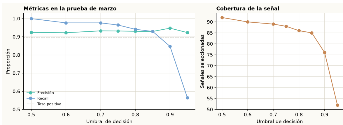
Figura 7.4: Métricas por umbral.
