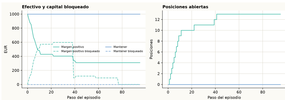
Figura 6.5: Trazas MARL.
