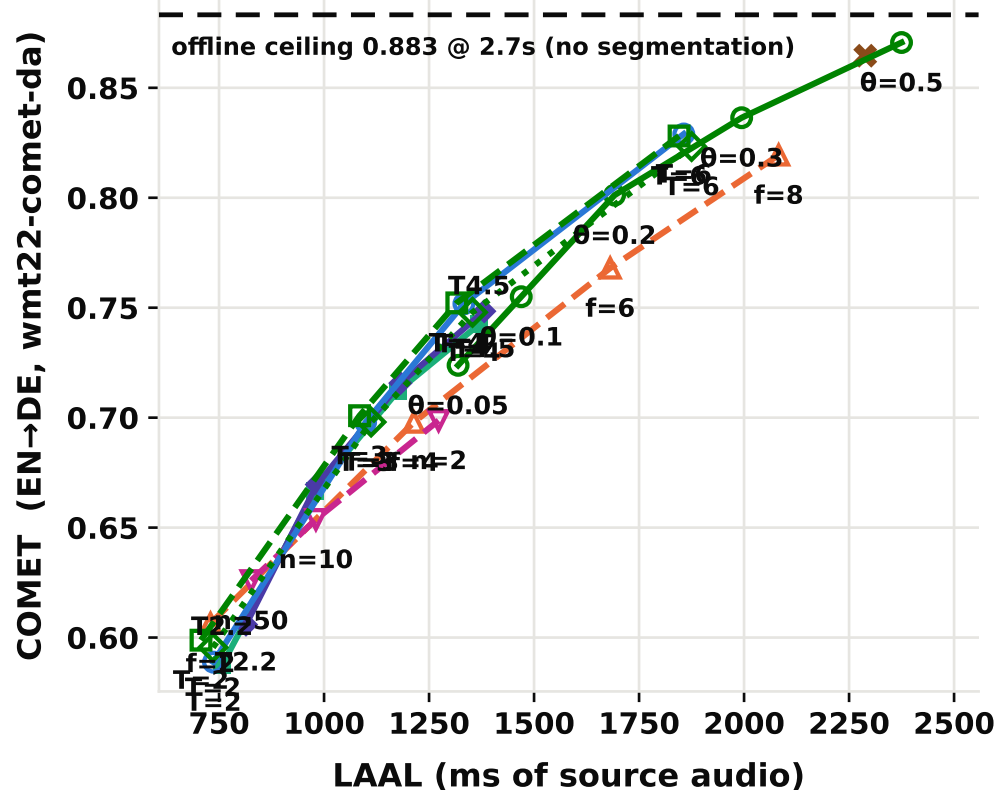
EN→DE
