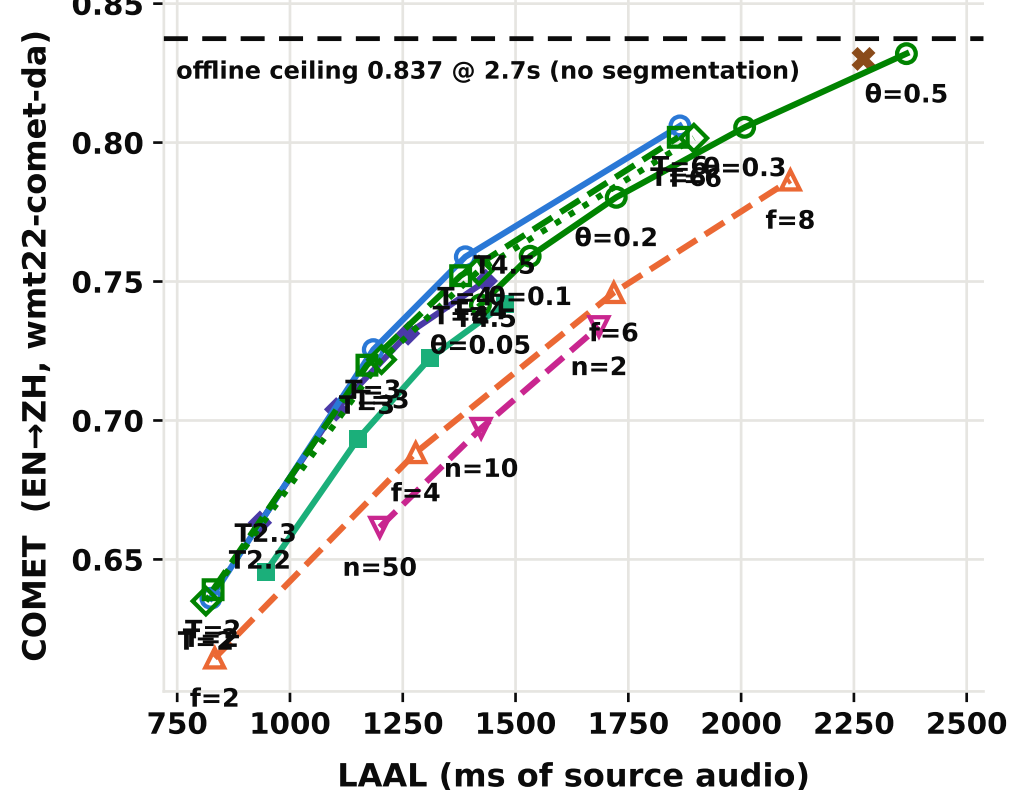
EN→ZH
