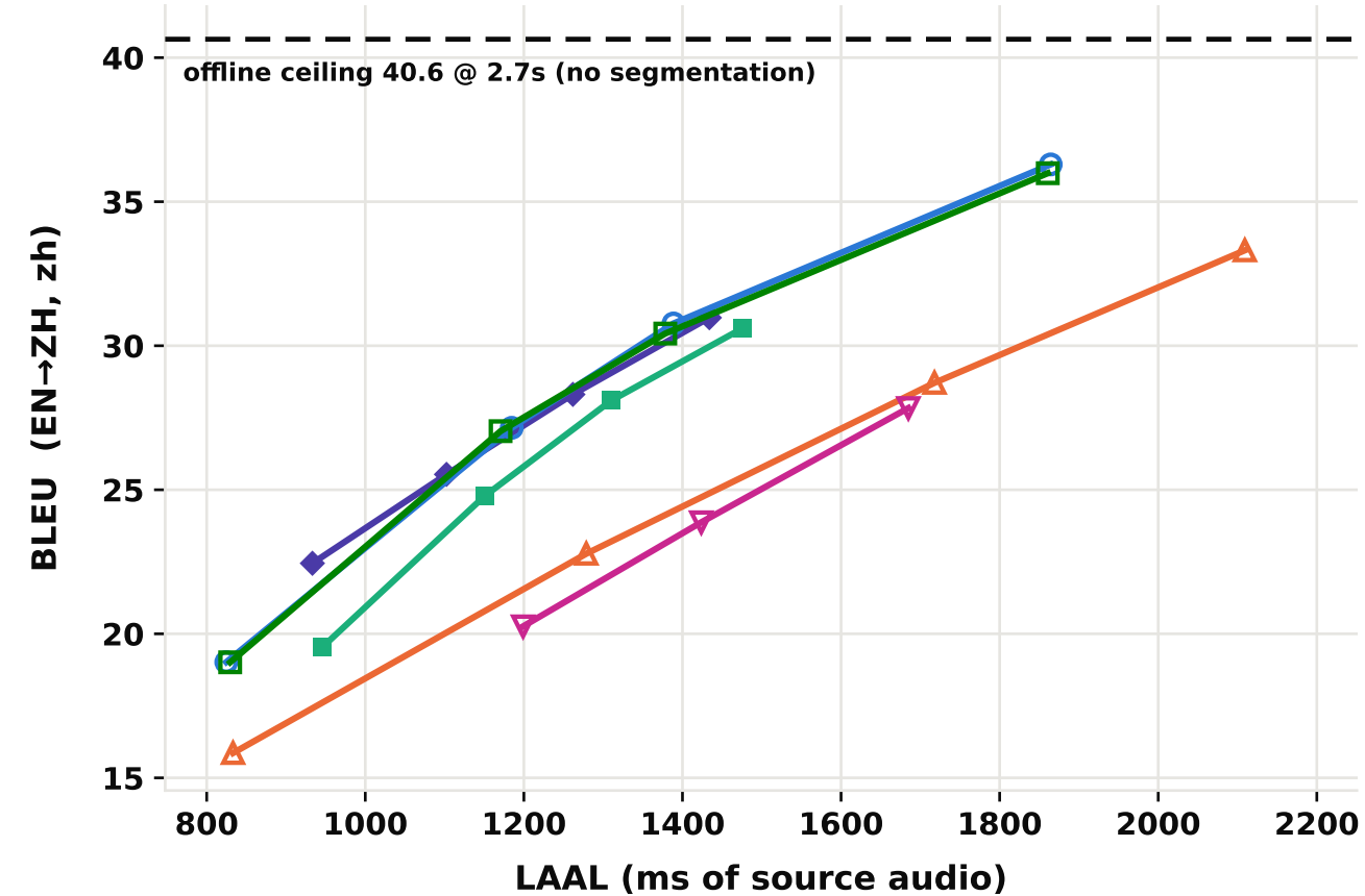
EN→ZH
