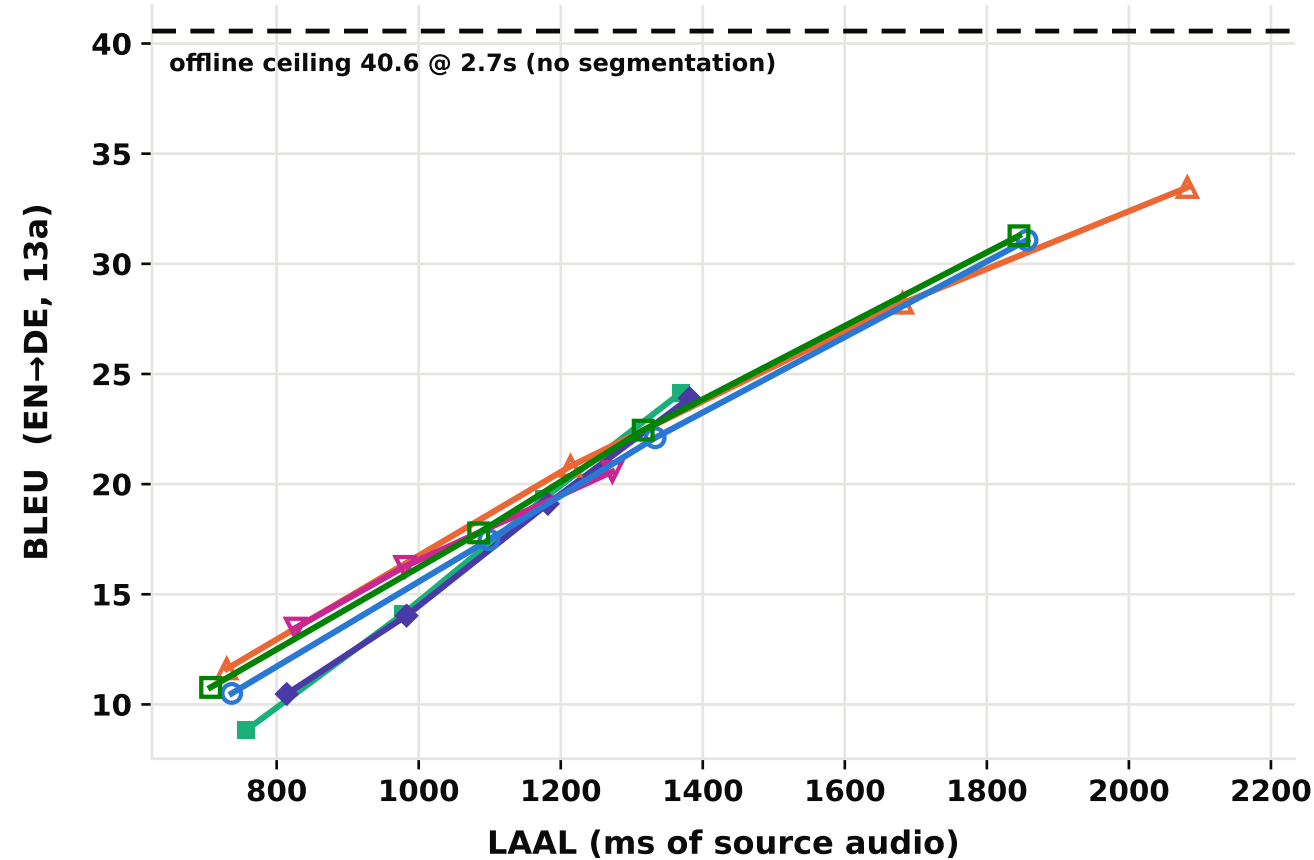
EN→DE
