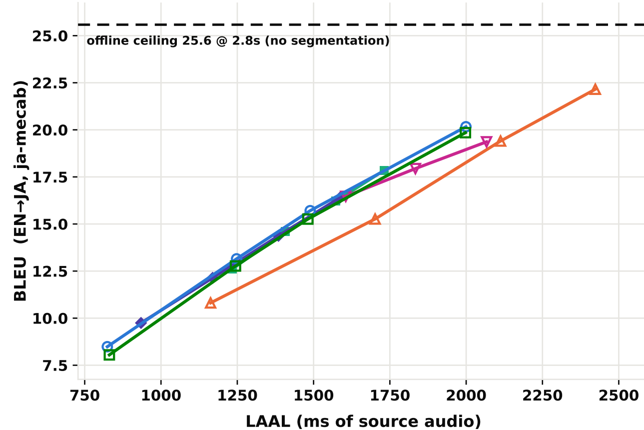
EN→JA
