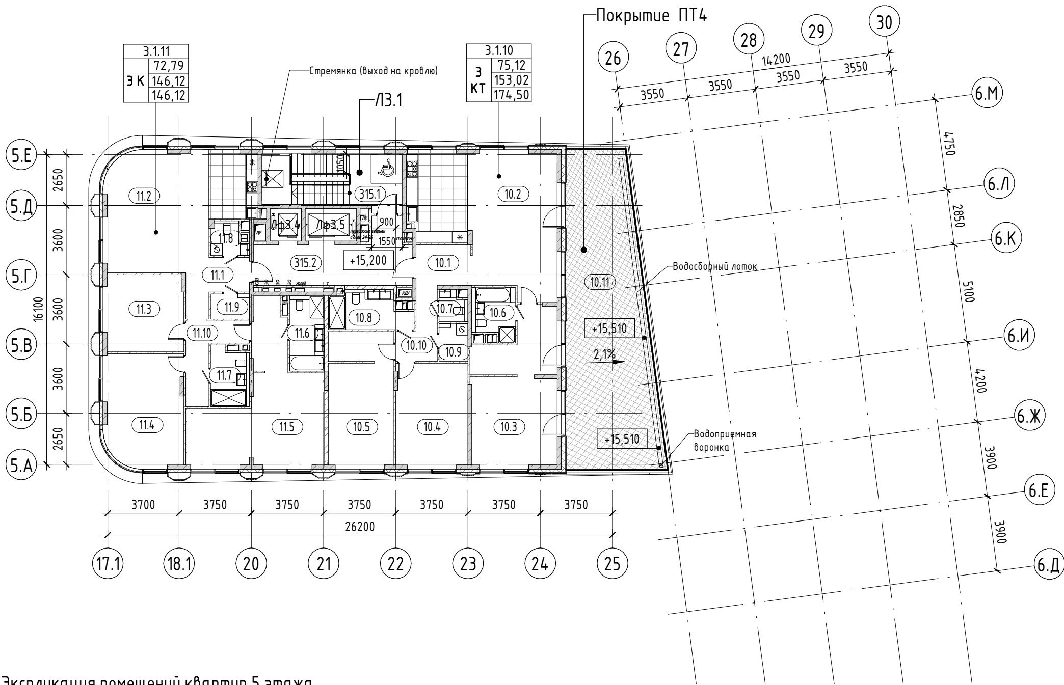
Экспликация помещений квартир 5 этажа (корпус 3.1)
