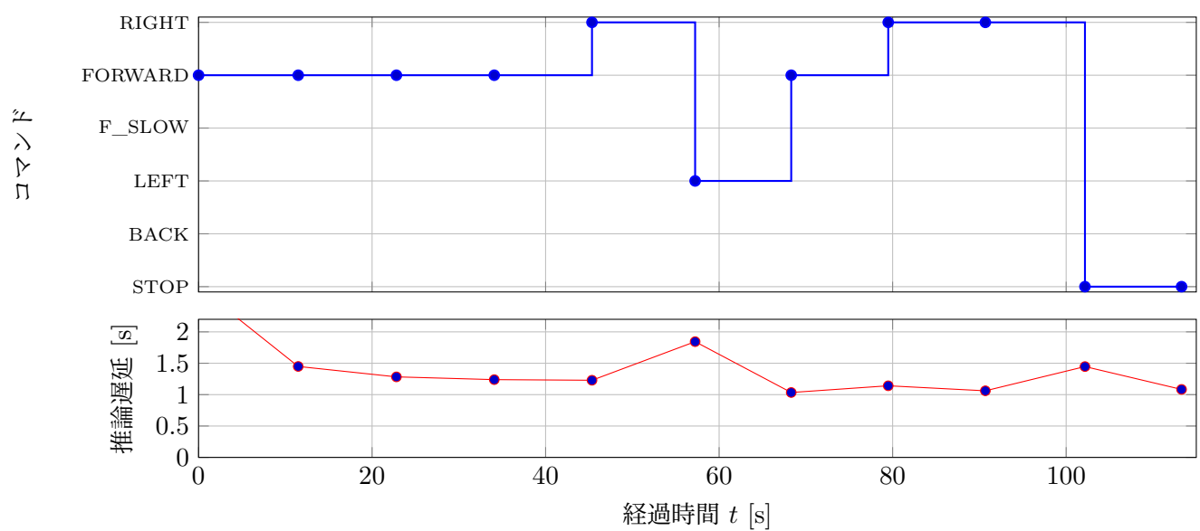
図 4.2 試行 A (照度 873 lx) 代表試行 (ログ ID: 172549, 通過で失敗) のコマンド系列と推論遅延。上段は時系列のコマンド (階段プロット), 下段は各ループの推論遅延。時間は最初の送信時刻を t = 0 とする。
