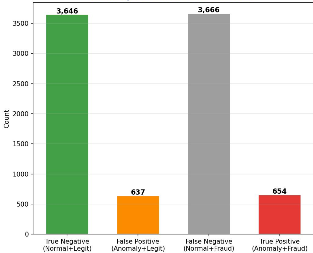
Anomaly Detection vs Actual Fraud
