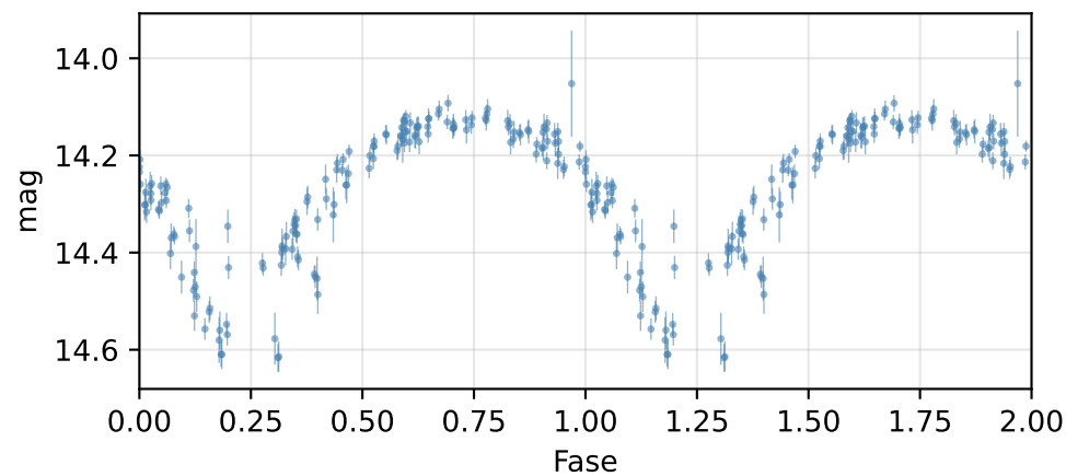
Curva de fase (P = 0.24452 d)
