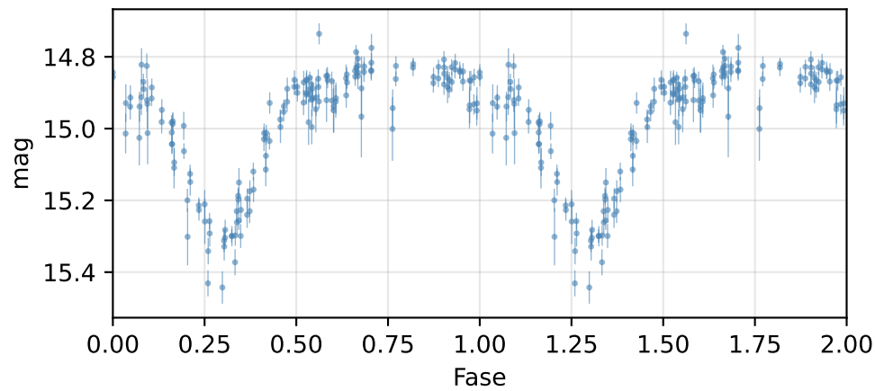
Curva de fase (P = 1.64433 d)
