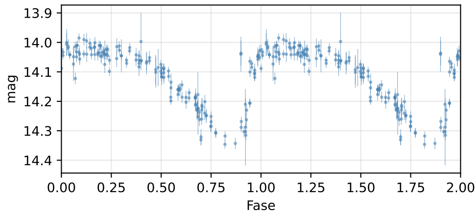
Curva de fase (P = 0.63166 d)
