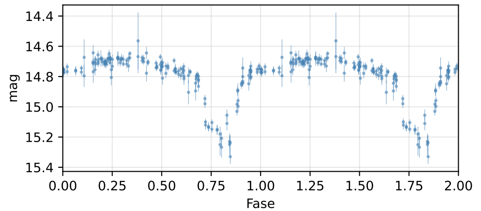
Curva de fase (P = 2.37266 d)
