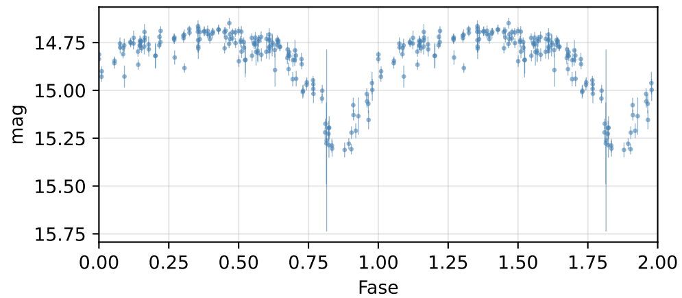
Curva de fase (P = 0.53269 d)
