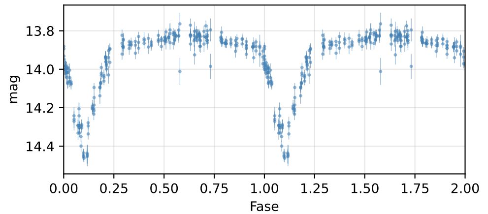
Curva de fase (P = 3.53705 d)
