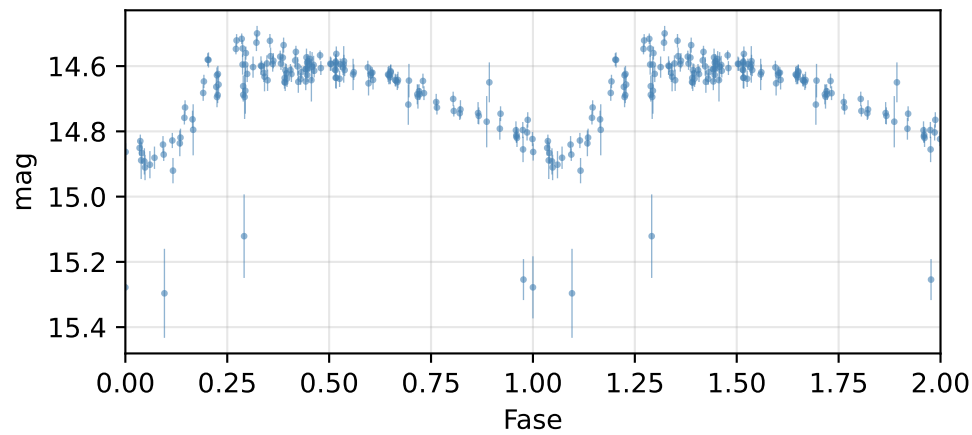
Curva de fase (P = 0.48692 d)
