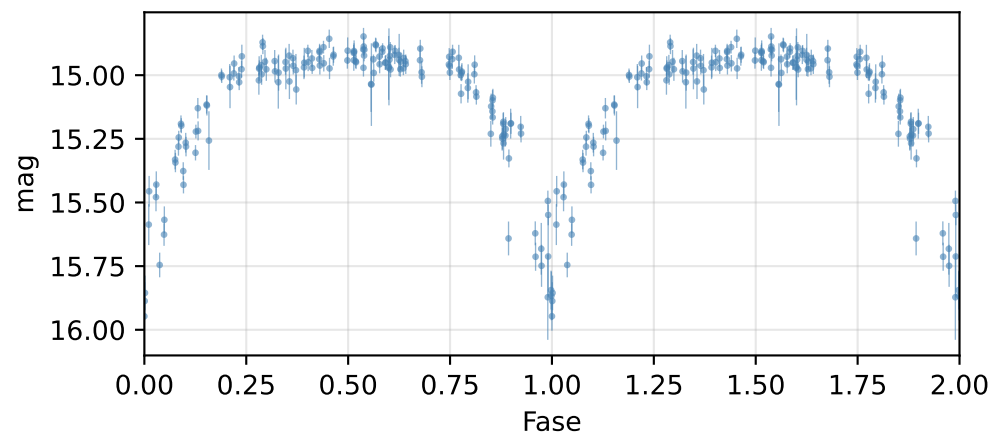
Curva de fase (P = 0.54546 d)
