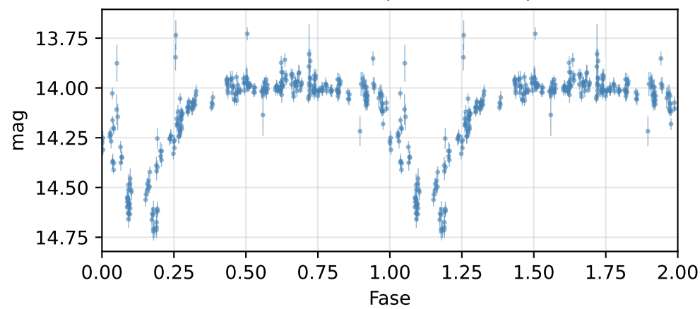
Curva de fase (P = 0.42192 d)
