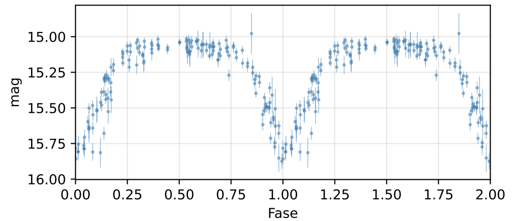
Curva de fase (P = 0.47402 d)
