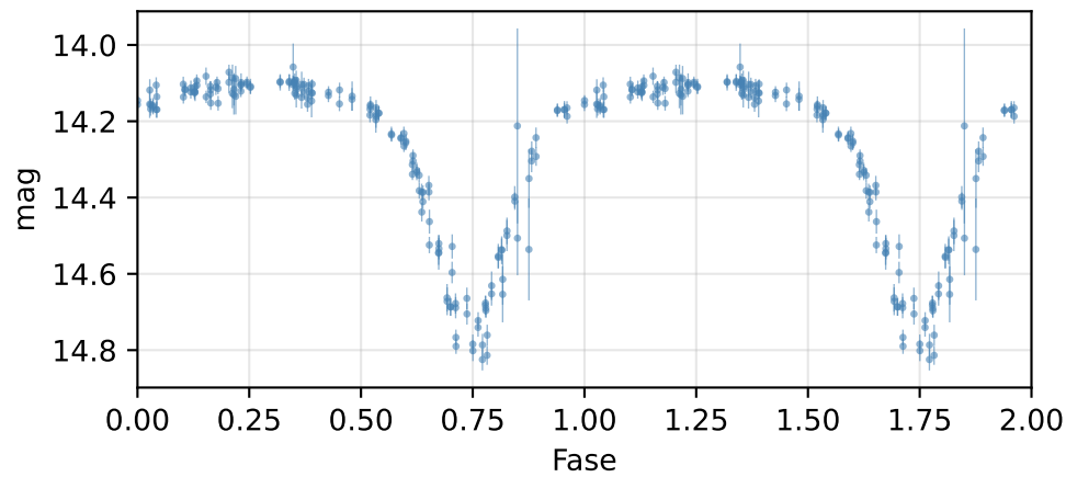
Curva de fase (P = 1.98187 d)
