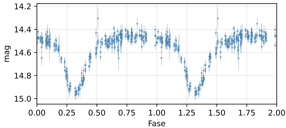
Curva de fase (P = 1.74796 d)
