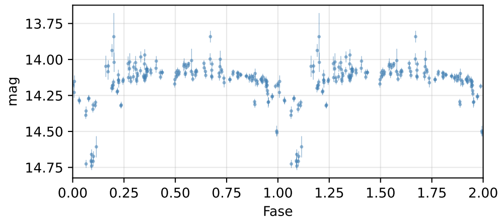
Curva de fase (P = 0.59288 d)
