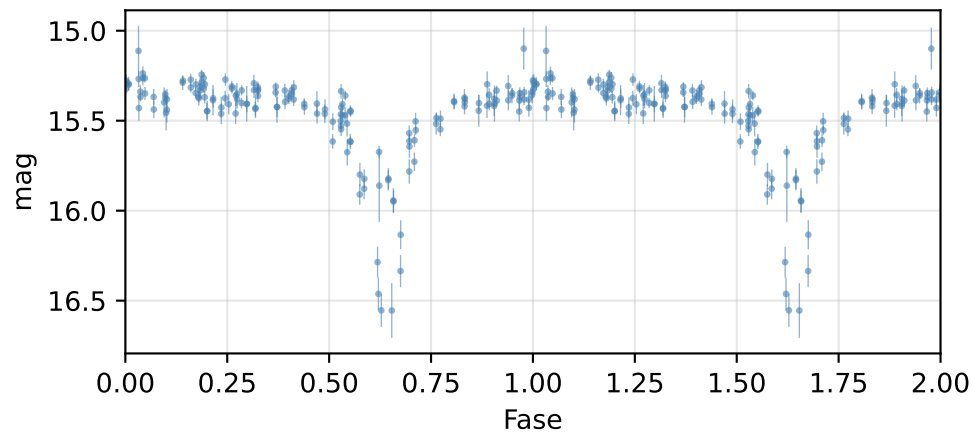
Curva de fase (P = 1.04045 d)
