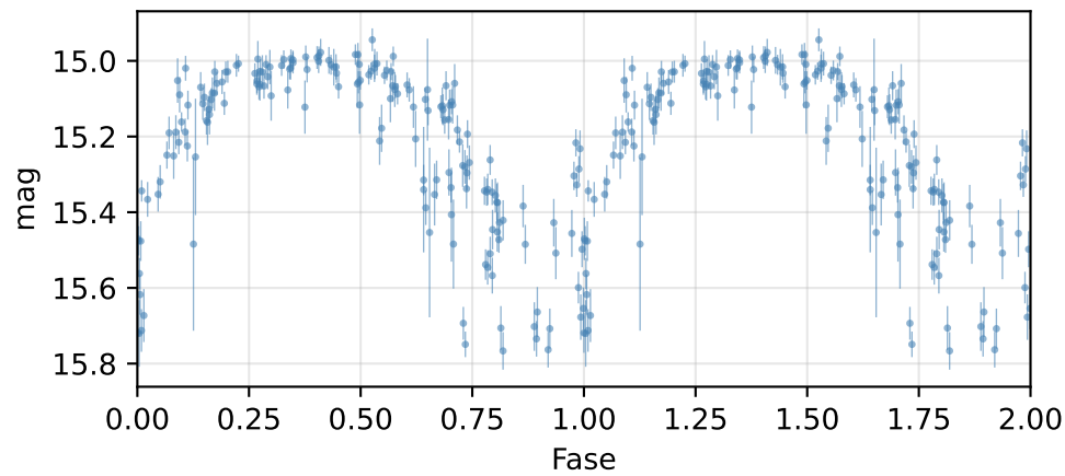
Curva de fase (P = 0.16887 d)
