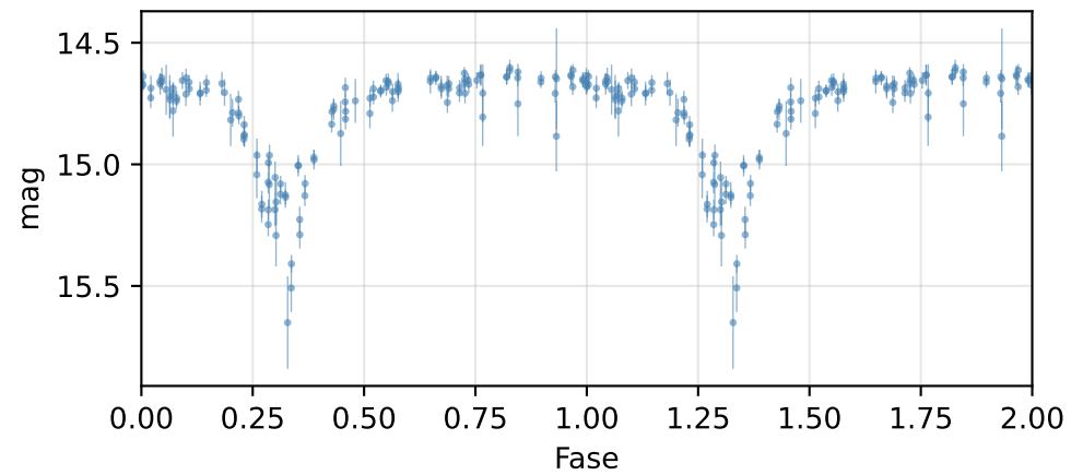
Curva de fase (P = 1.08863 d)
