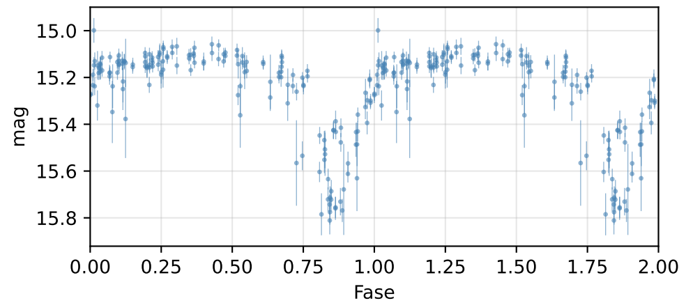
Curva de fase (P = 1.08737 d)
