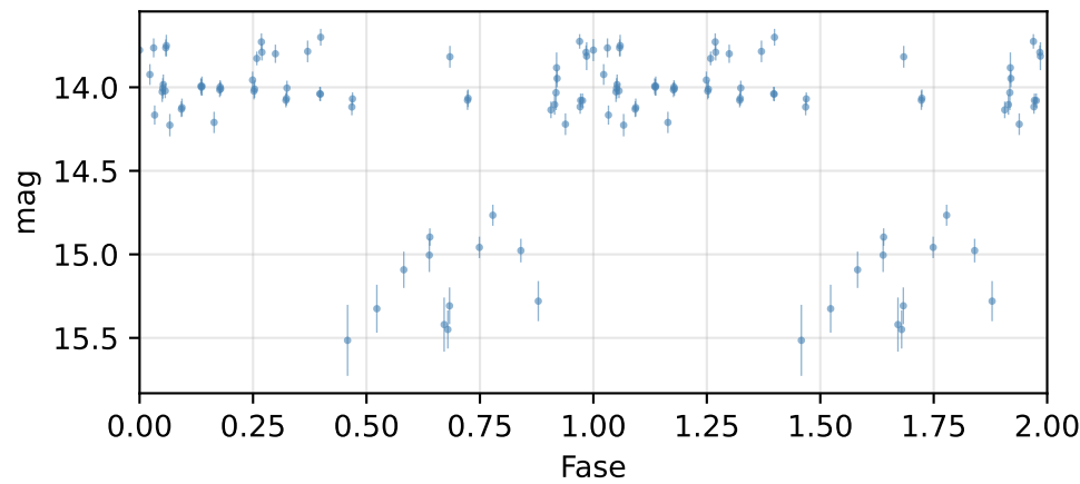
Curva de fase (P = 0.35363 d)
