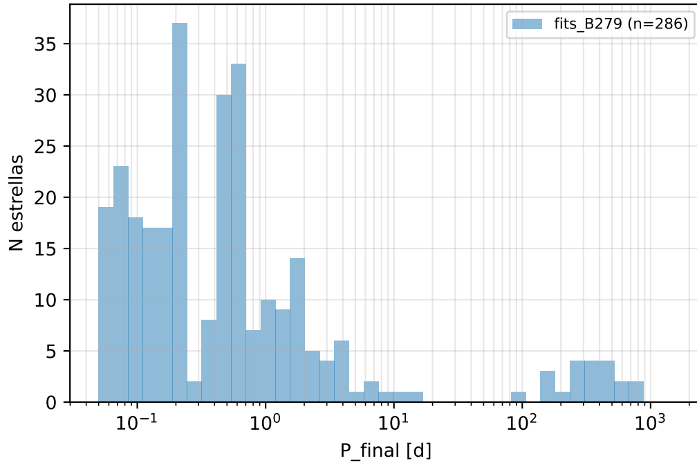
Distribucion de P_final
