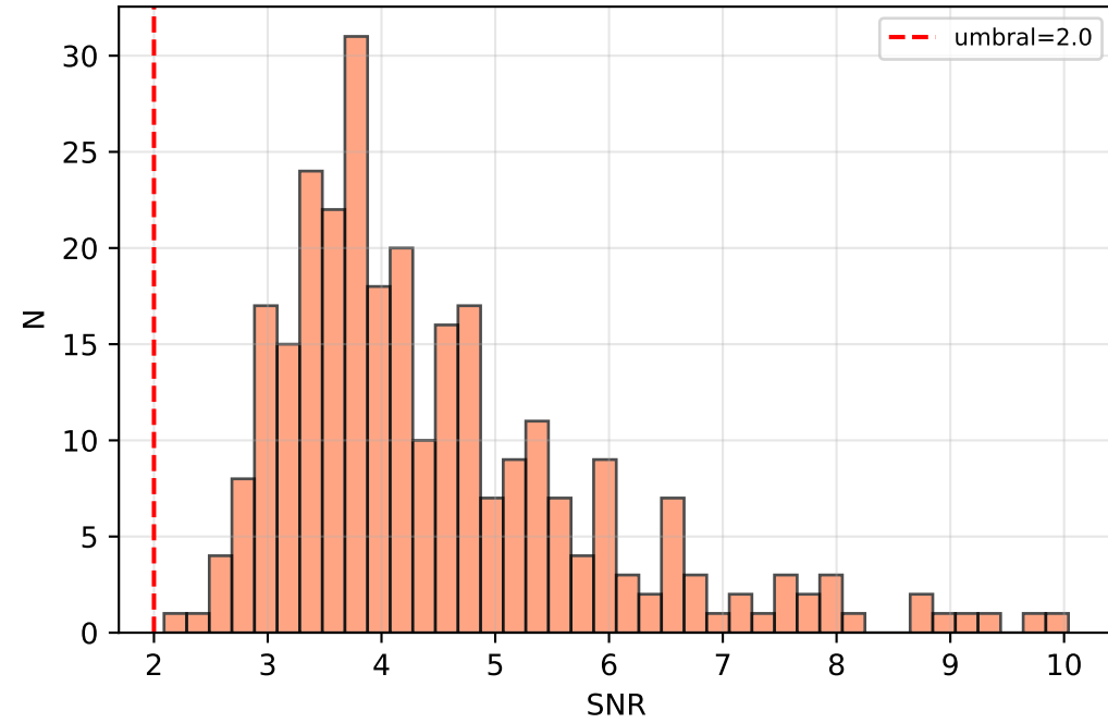
Distribucion de SNR
