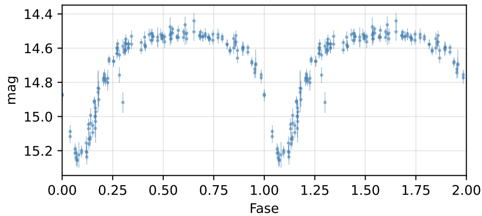
Curva de fase (P = 1.63759 d)
