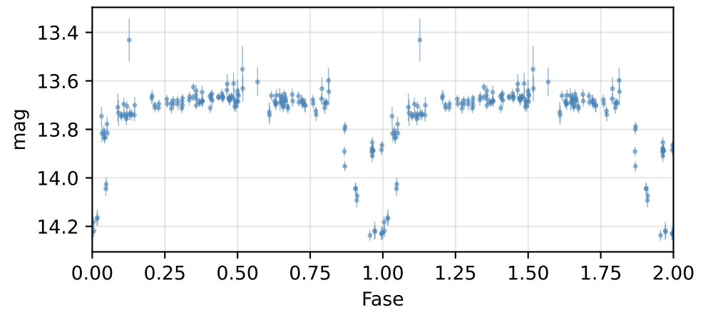
Curva de fase (P = 0.64727 d)
