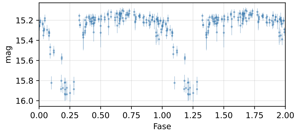
Curva de fase (P = 1.11792 d)
