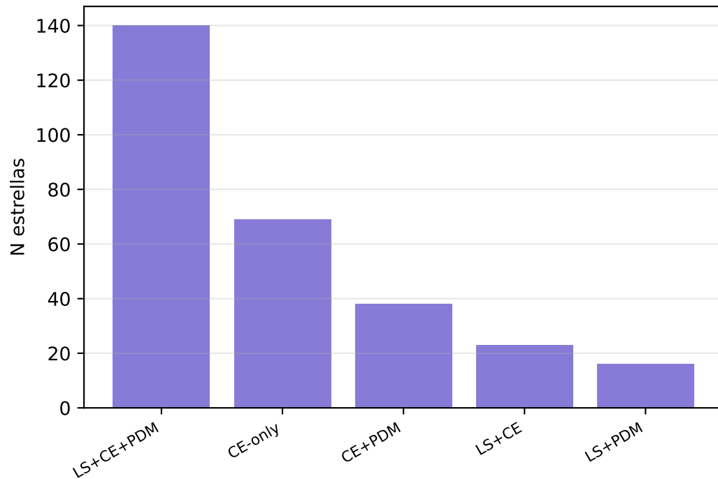
Consenso entre metodos
