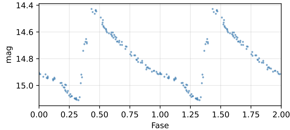
Curva de fase (P = 0.52317 d)
