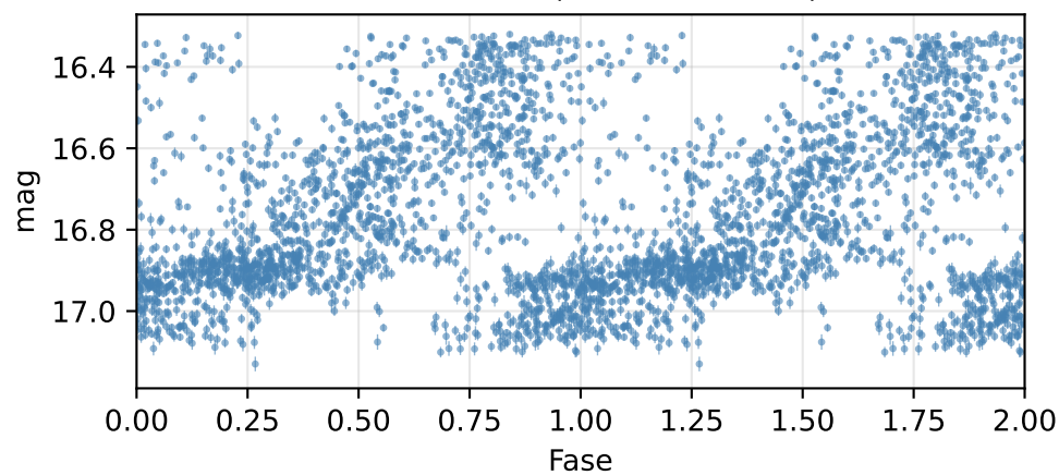
Curva de fase (P = 484.17130 d)
