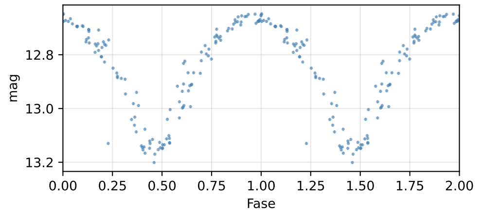
Curva de fase (P = 0.21941 d)
