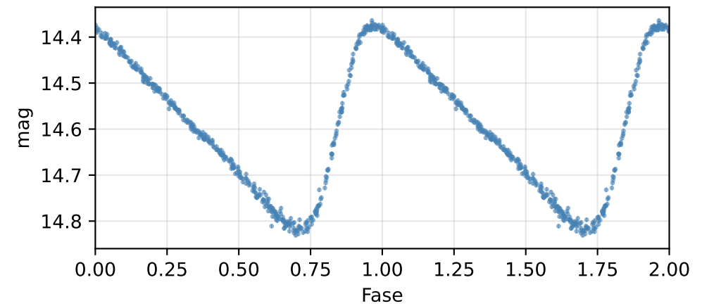
Curva de fase (P = 5.10627 d)
