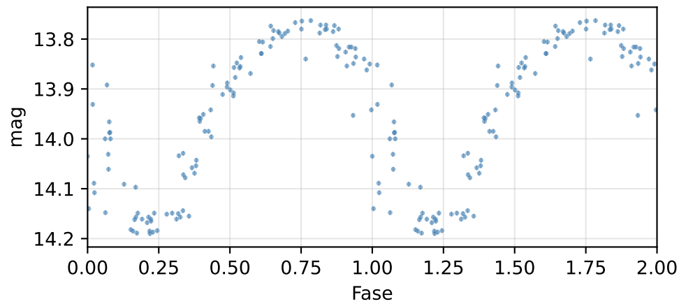
Curva de fase (P = 0.14224 d)
