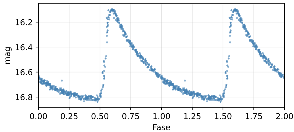
Curva de fase (P = 1.32592 d)
