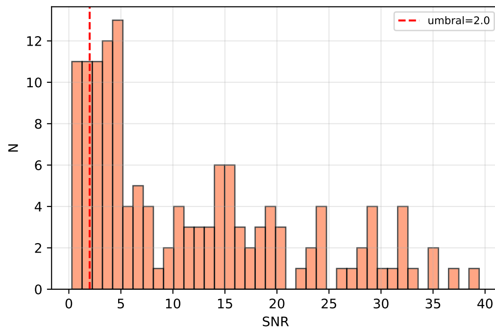
Distribucion de SNR
