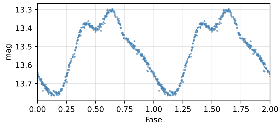
Curva de fase (P = 10.91709 d)
