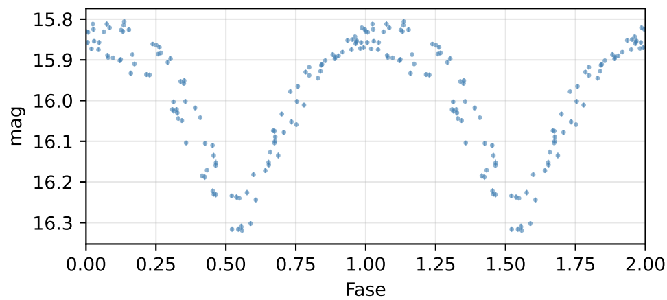
Curva de fase (P = 0.15949 d)
