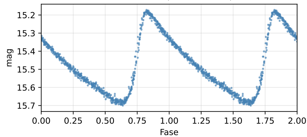
Curva de fase (P = 2.77817 d)
