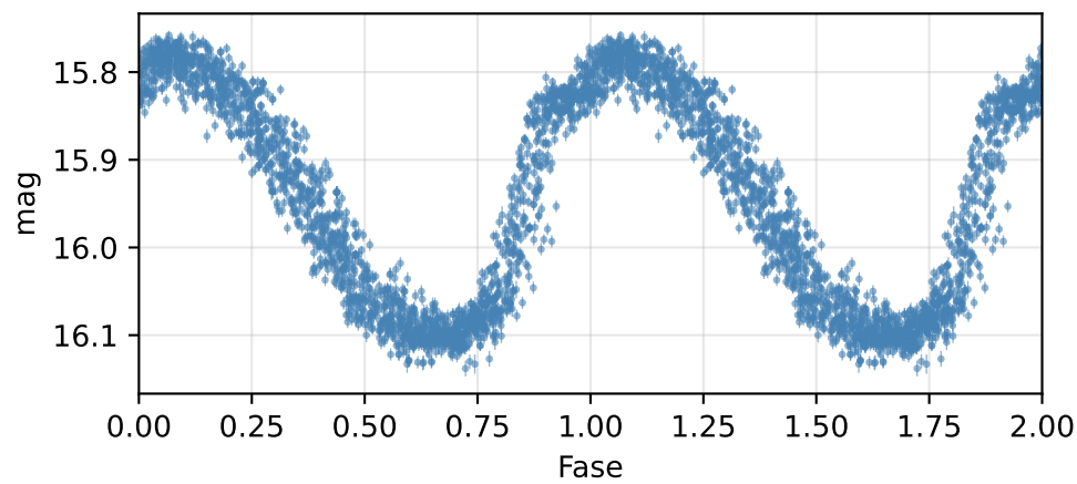
Curva de fase (P = 0.27538 d)
