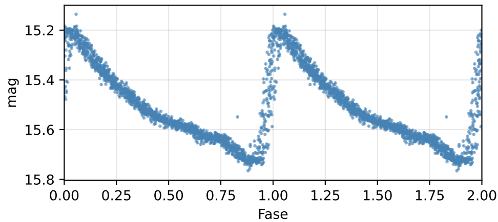
Curva de fase (P = 0.47318 d)
