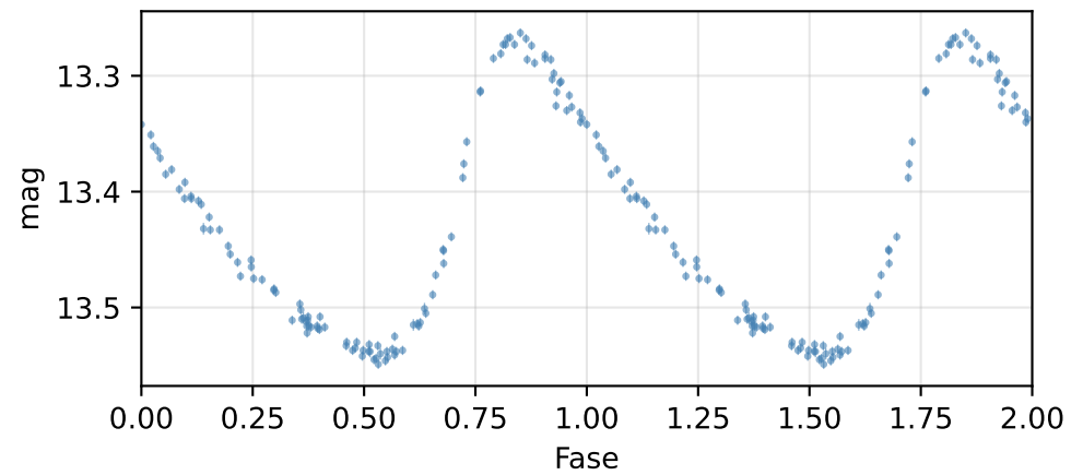
Curva de fase (P = 0.09863 d)
