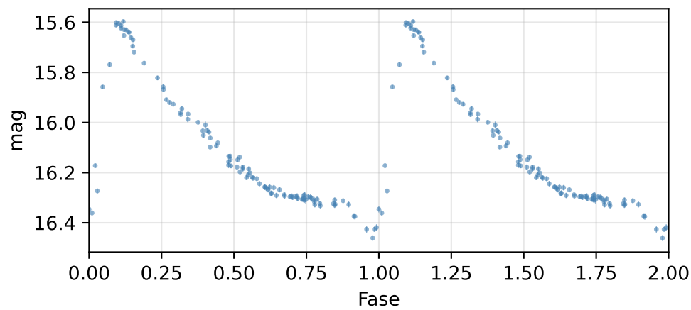
Curva de fase (P = 0.49240 d)
