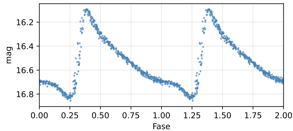
Curva de fase (P = 1.76137 d)
