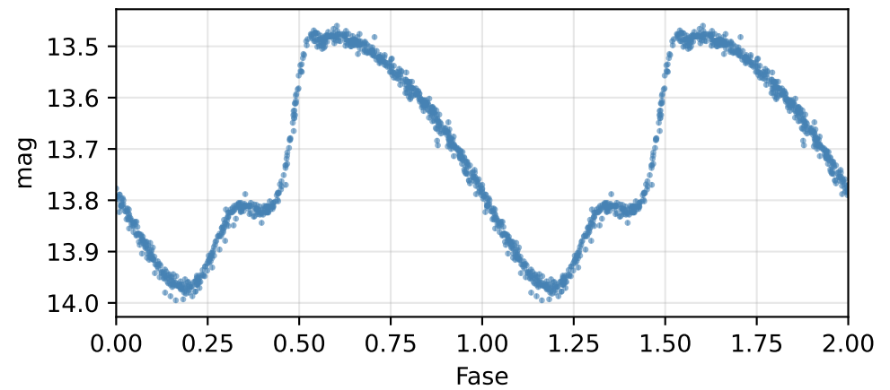
Curva de fase (P = 12.72091 d)
