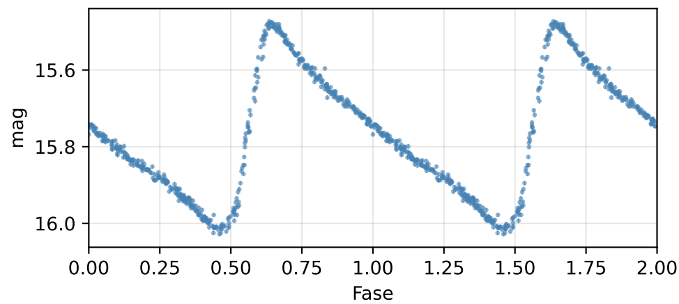
Curva de fase (P = 3.14110 d)
