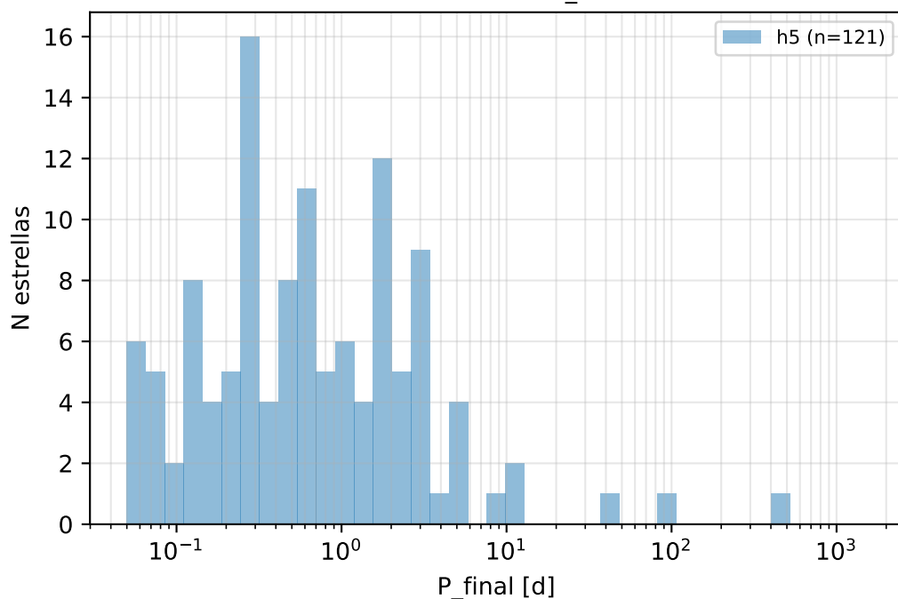
Consenso entre metodos
