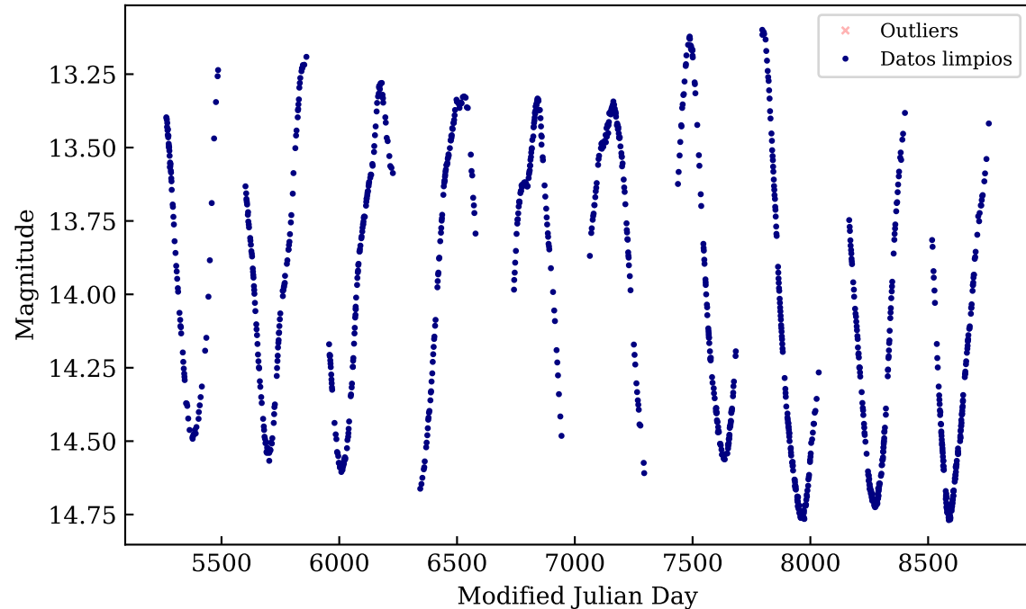
OGLE-BLG-LPV-004280
