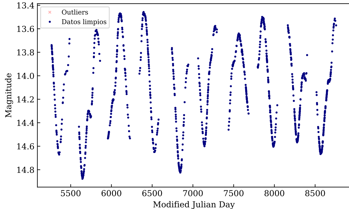
OGLE-BLG-LPV-003977
