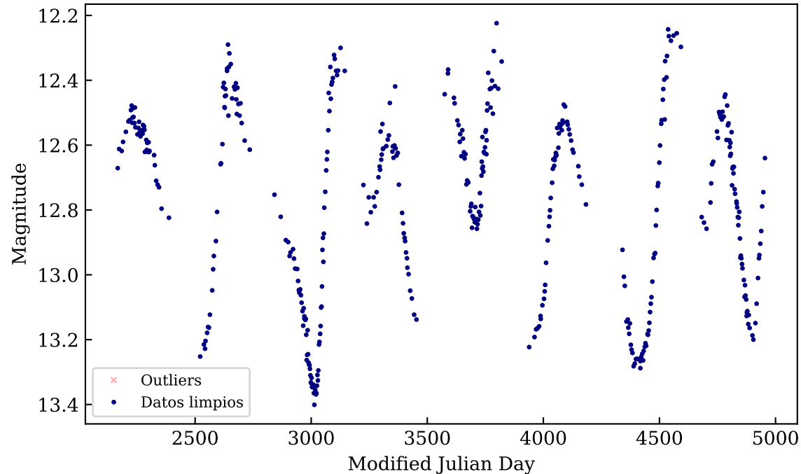
OGLE-LMC-LPV-11378
