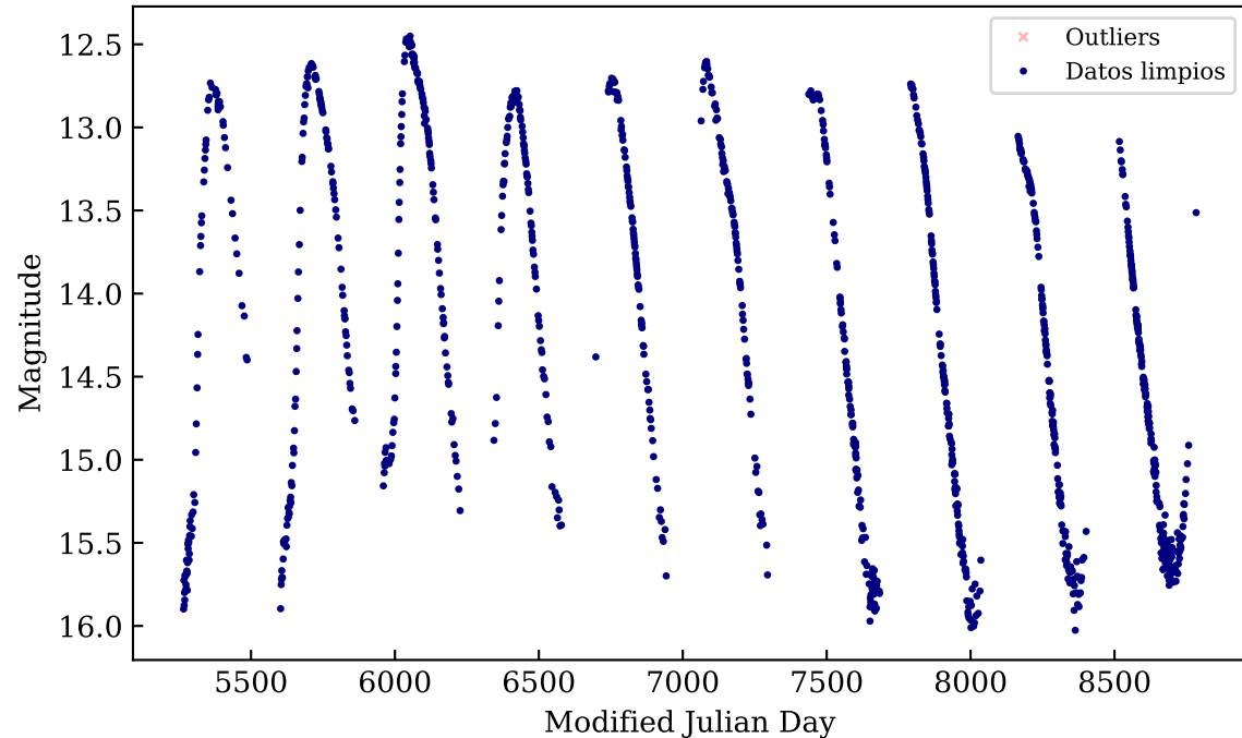
OGLE-BLG-LPV-005621
