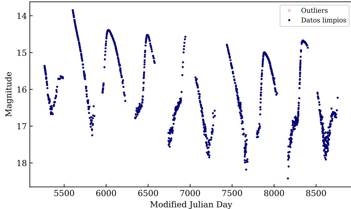
OGLE-BLG-LPV-002259
