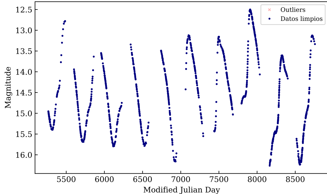
OGLE-BLG-LPV-002045
