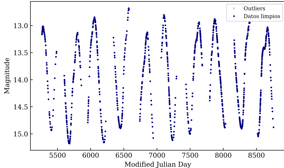
OGLE-BLG-LPV-002911
