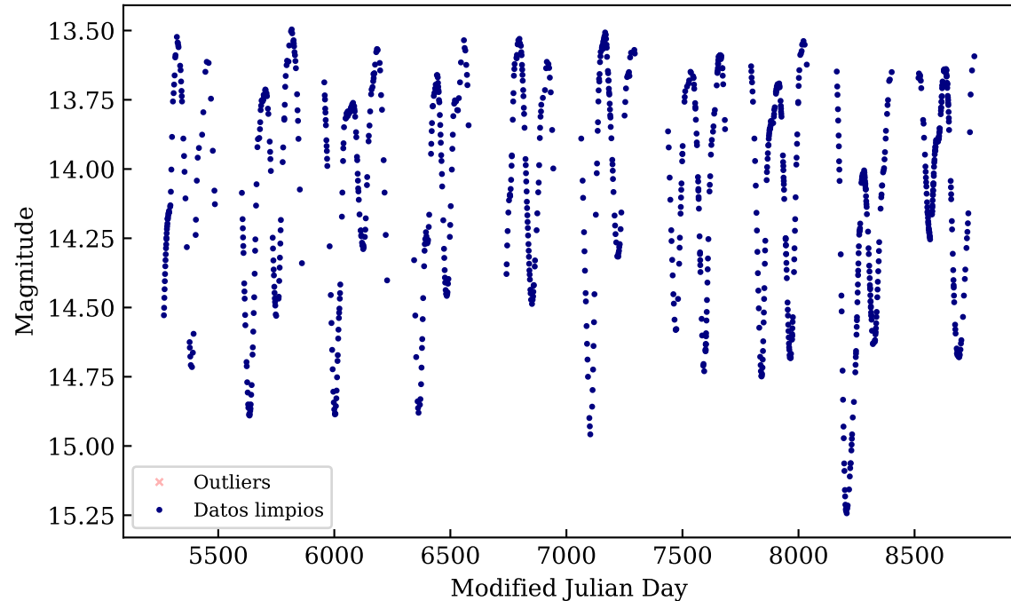
OGLE-BLG-LPV-003126
