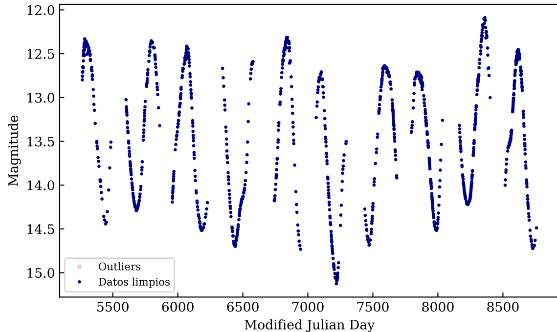
OGLE-BLG-LPV-005152
