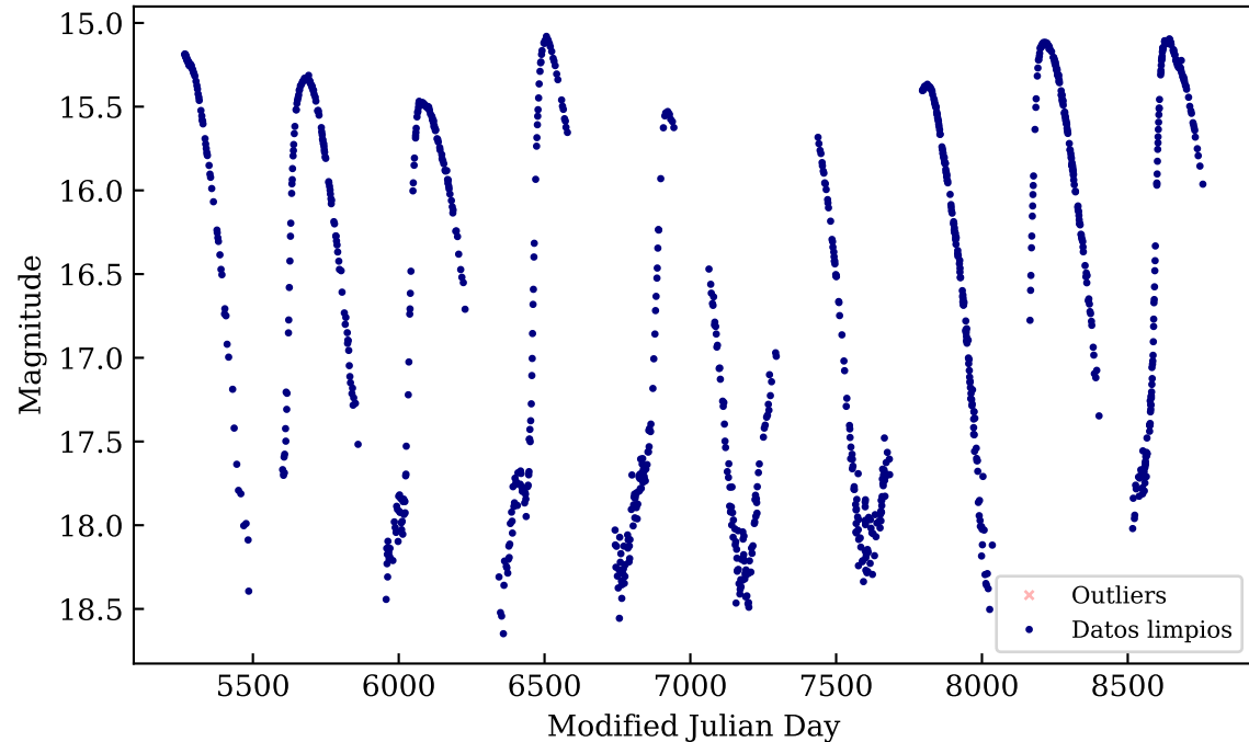
OGLE-BLG-LPV-004009
