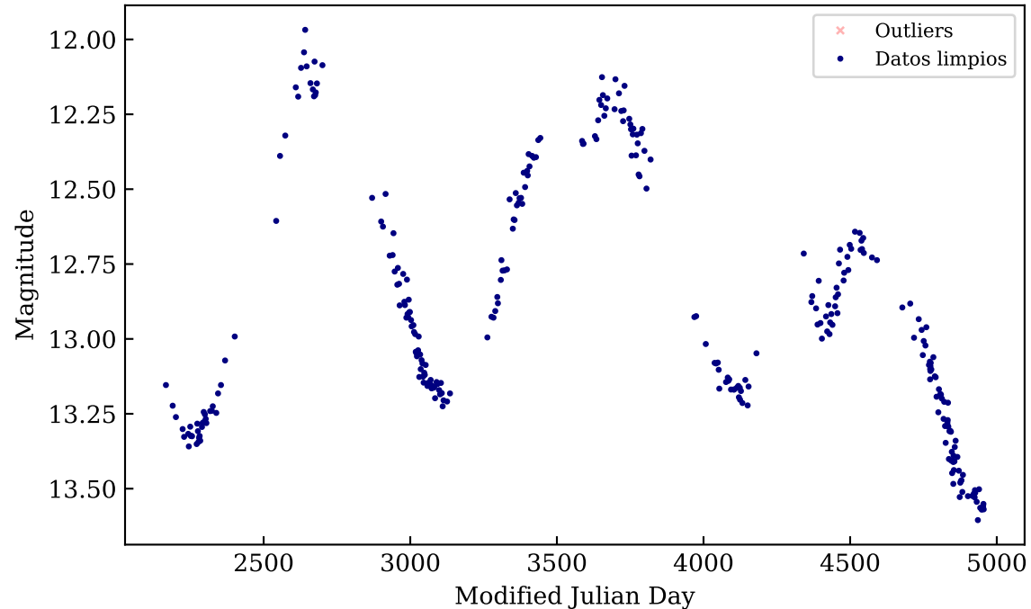
OGLE-LMC-LPV-06819
