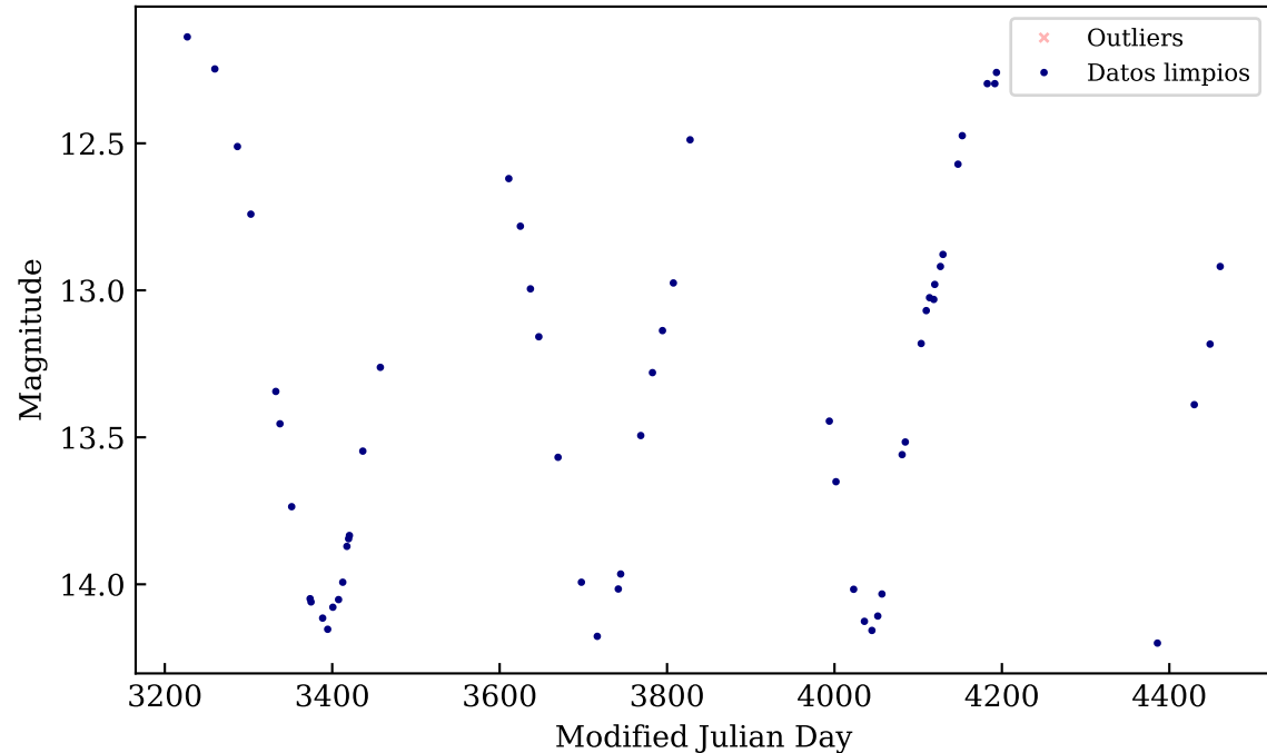
OGLE-LMC-LPV-09008
