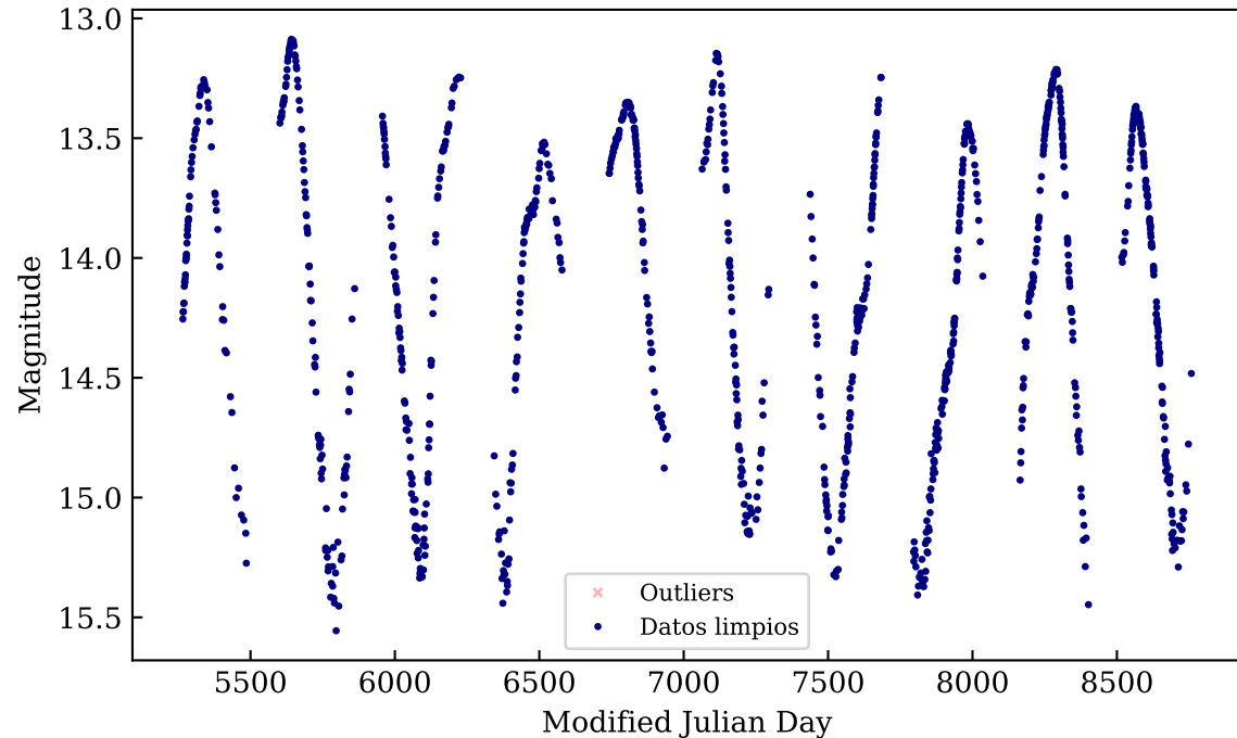
OGLE-BLG-LPV-003676
