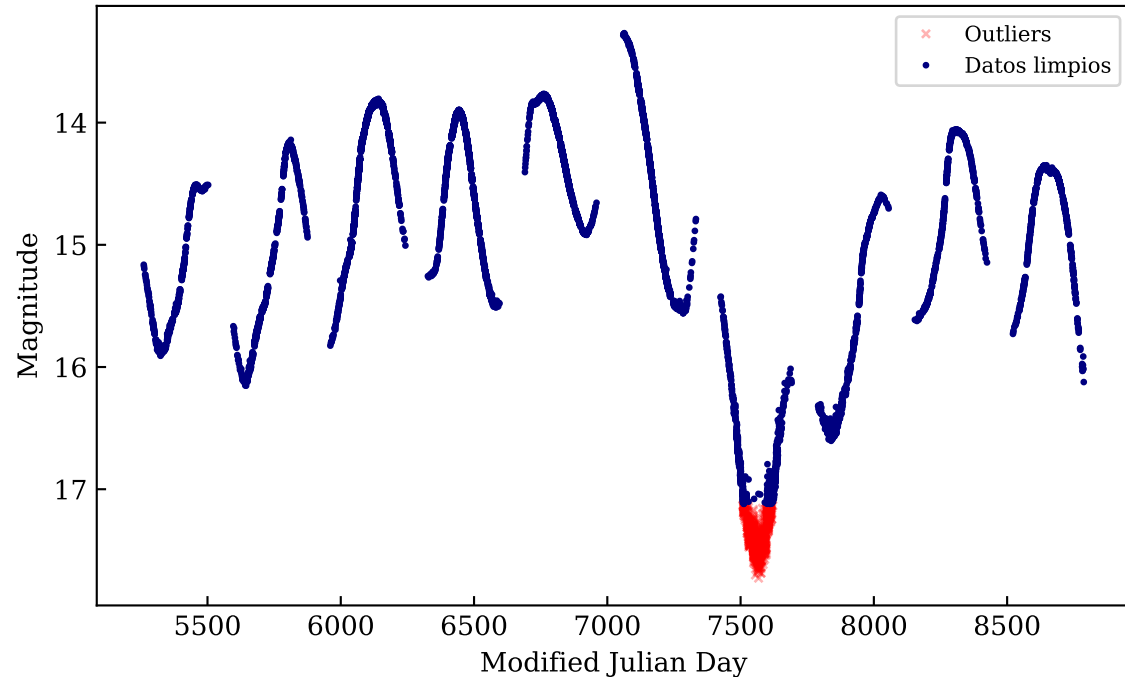
OGLE-BLG-LPV-176699
