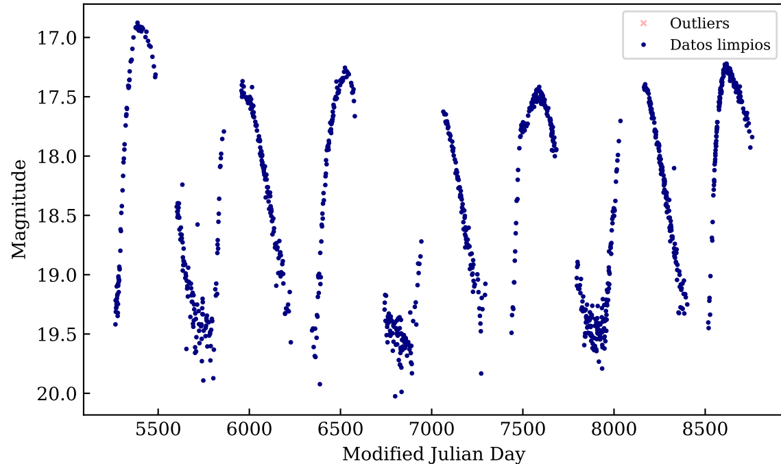
OGLE-BLG-LPV-002162
