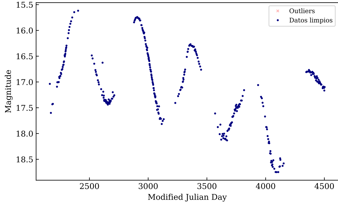
OGLE-LMC-LPV-00449
