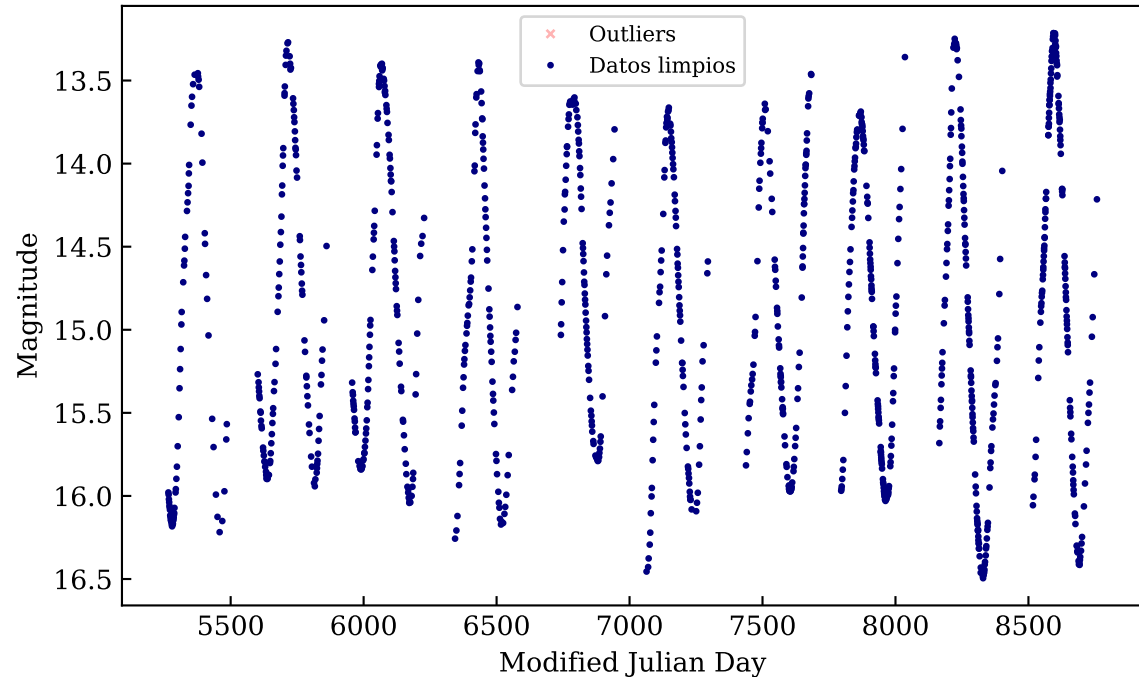
OGLE-BLG-LPV-003858
