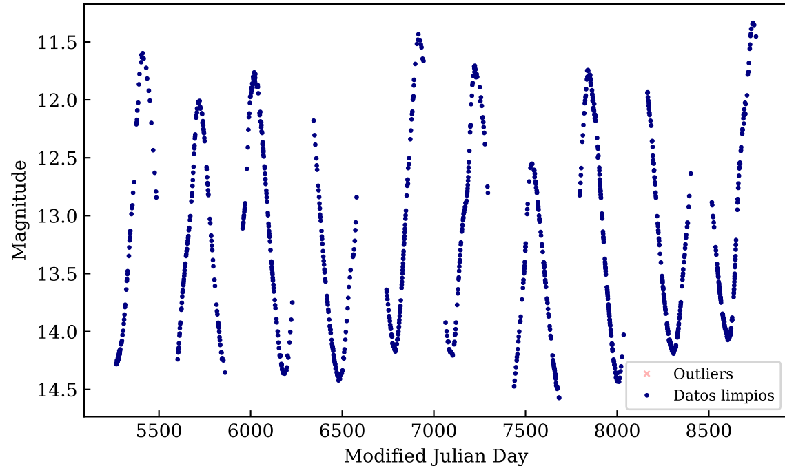
OGLE-BLG-LPV-003256
