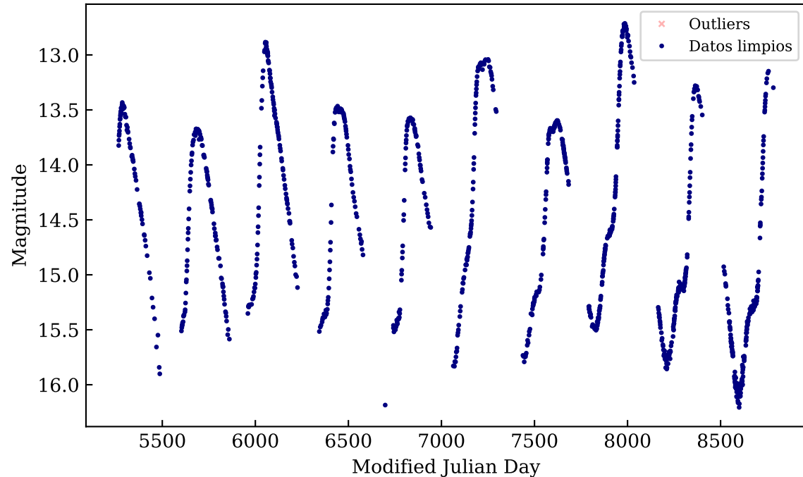
OGLE-BLG-LPV-005545
