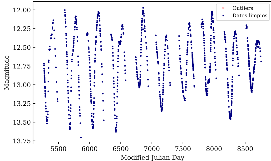
OGLE-BLG-LPV-003330
