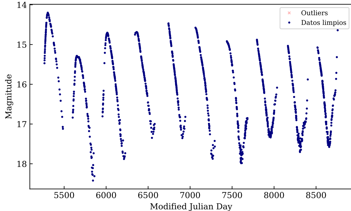
OGLE-BLG-LPV-004082
