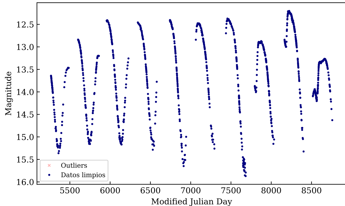
OGLE-BLG-LPV-004248
