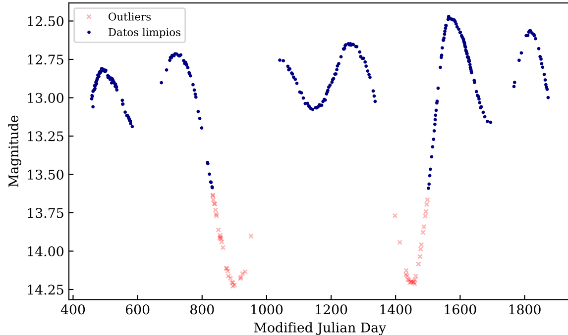
OGLE-LMC-LPV-25968
