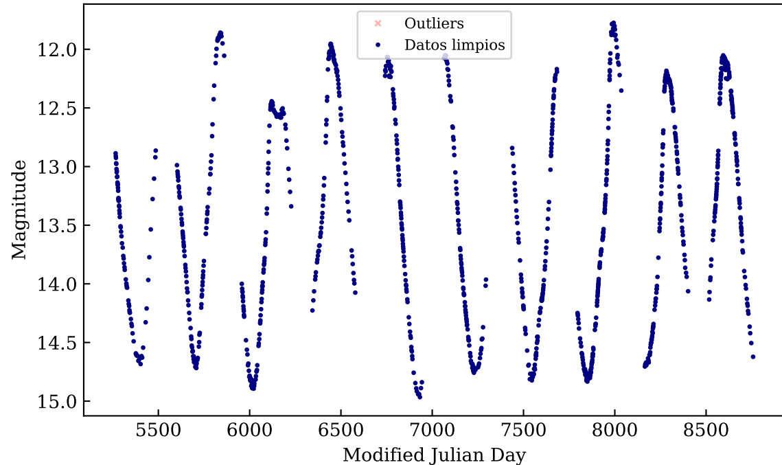
OGLE-BLG-LPV-005264
