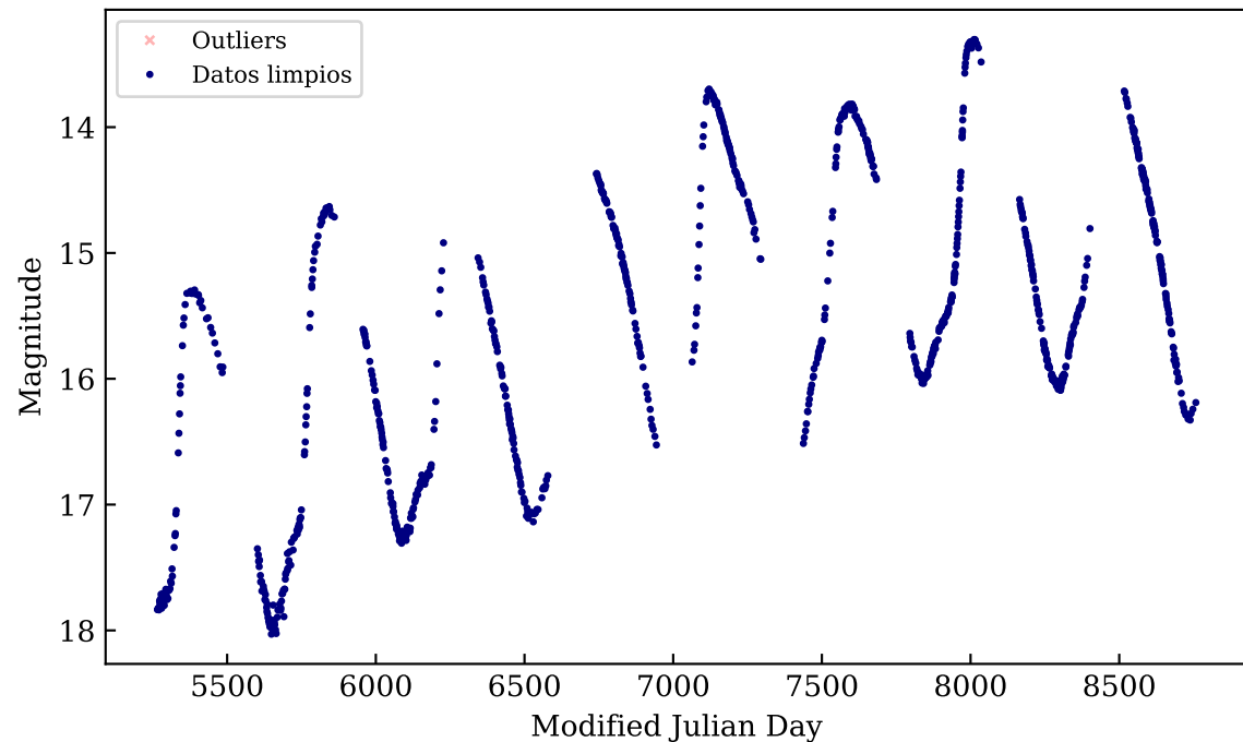
OGLE-BLG-LPV-002778
