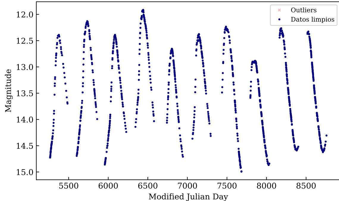
OGLE-BLG-LPV-004623
