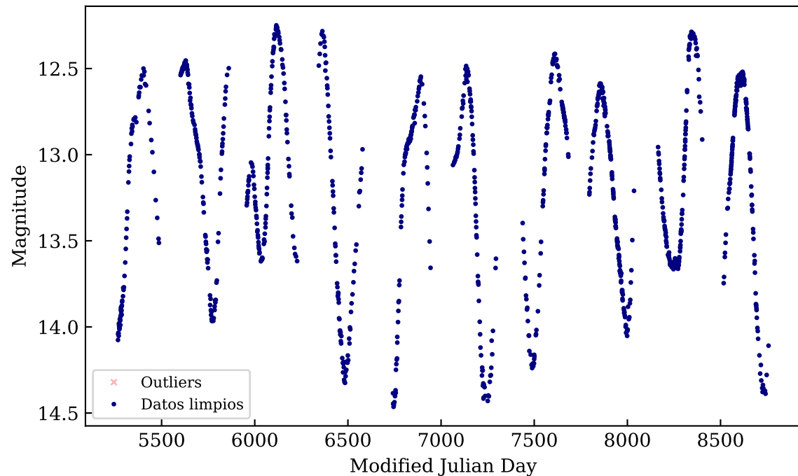
OGLE-BLG-LPV-002883
