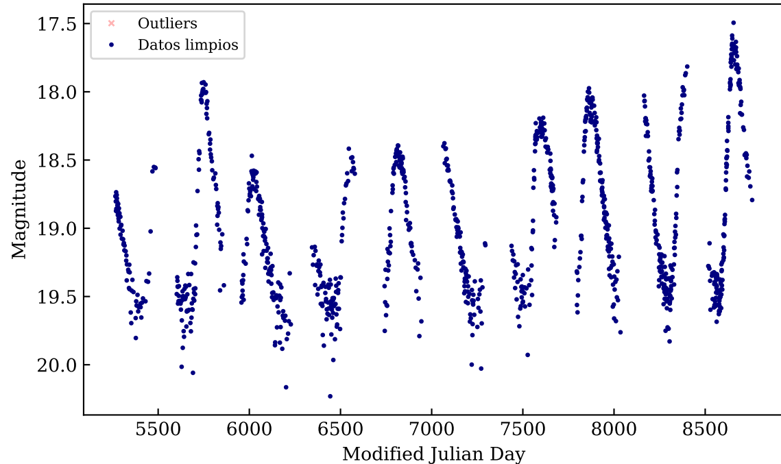
OGLE-BLG-LPV-003531
