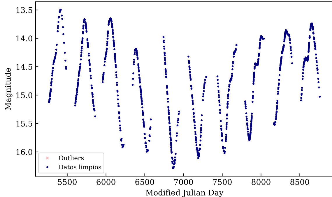
OGLE-BLG-LPV-004020
