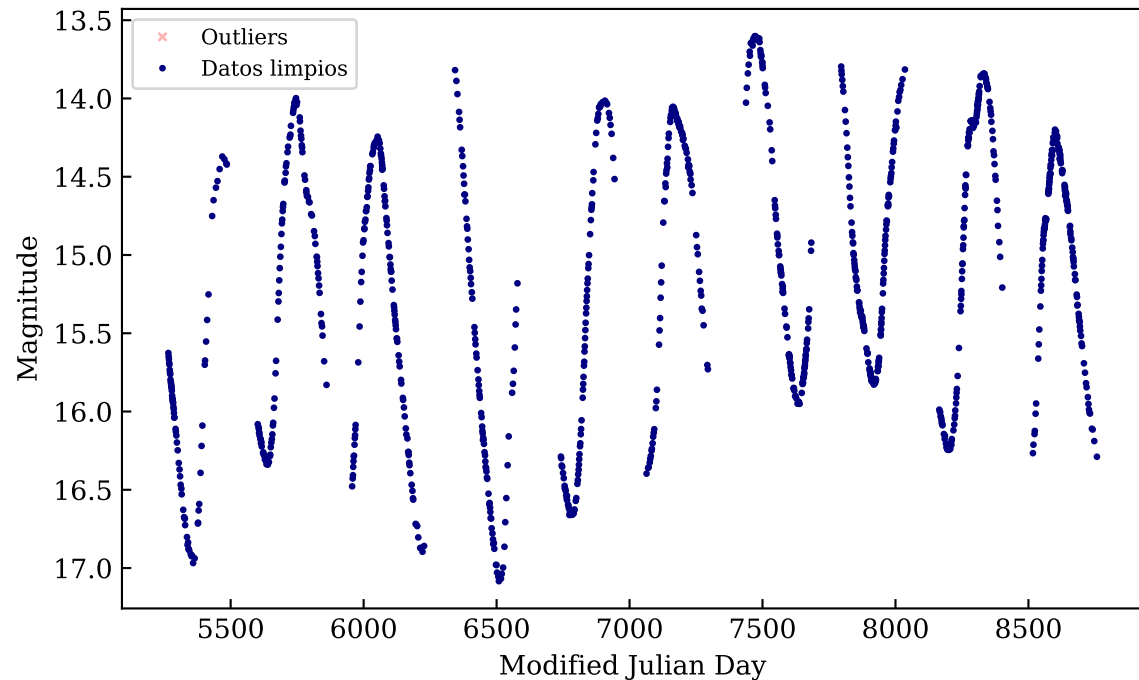
OGLE-BLG-LPV-004630
