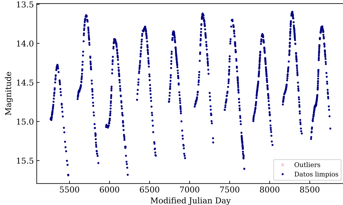
OGLE-BLG-LPV-004489
