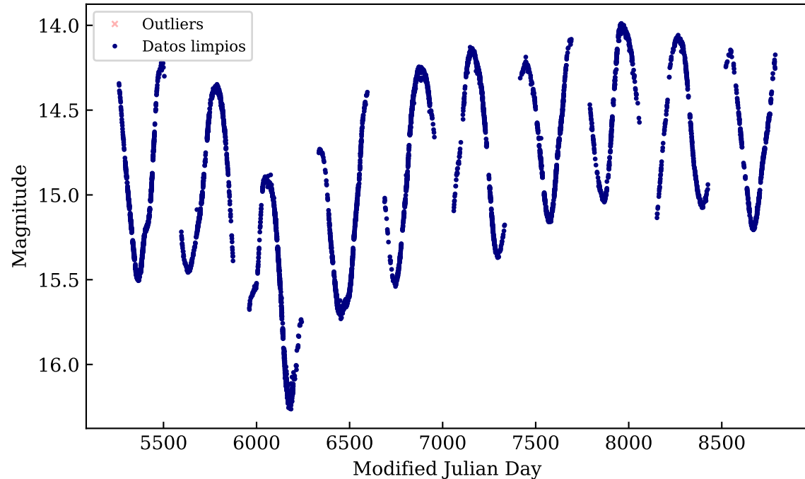
OGLE-BLG-LPV-124320
