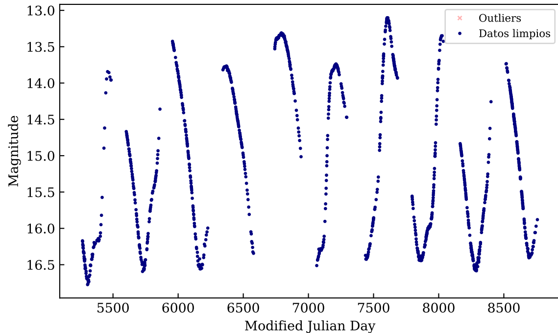
OGLE-BLG-LPV-002215
