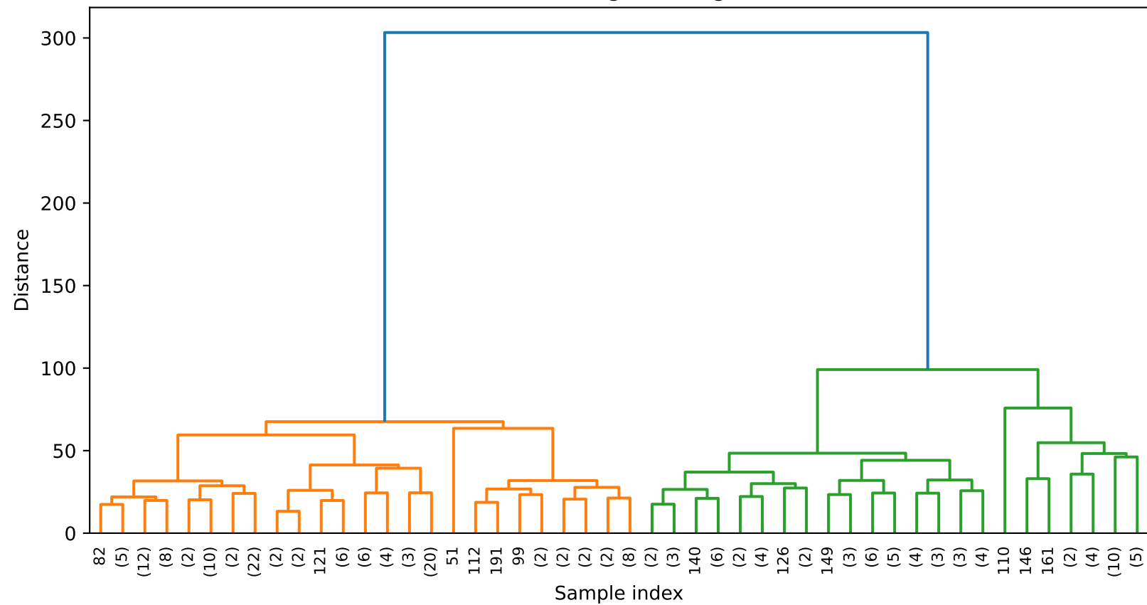
Hierarchical Clustering Dendrogram (Subset)
