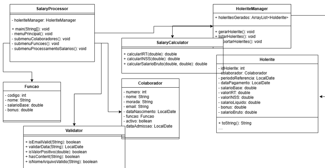
Figura 5 - Diagrama de classes do programa
