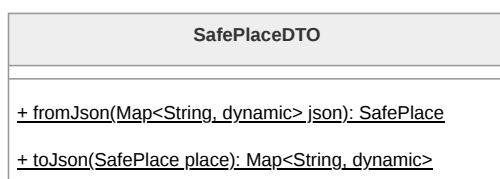
Figura 59: Diagramma della classe SafePlaceDTO
