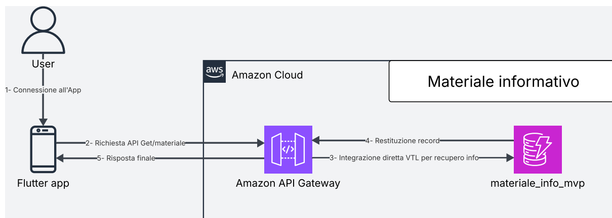
Figura 100: Architettura G moduli Materiale Informativo
