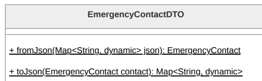
Figura 97: Diagramma della classe EmergencyContactDTO
