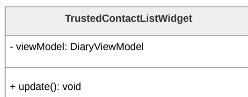
Figura 44: Diagramma della classe TrustedContactListWidget
