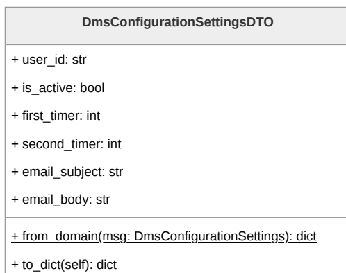
Figura 174: Diagramma della classe DmsConfigurationSettingsDTO
