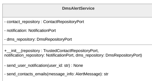
Figura 185: Diagramma della classe DmsAlertService
