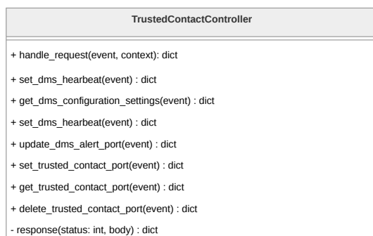
Figura 175: Diagramma della classe TrustedContactController
