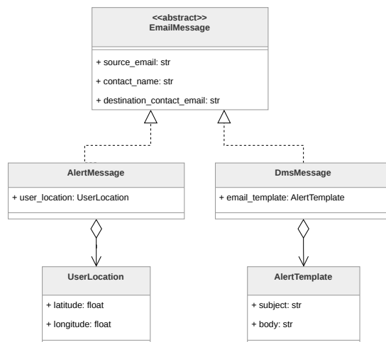
Figura 174: Diagramma della classe EmailMessage
