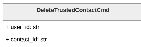
Figura 171: Diagramma della classe DeleteTrustedContactCmd
