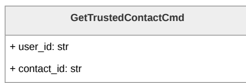
Figura 170: Diagramma della classe GetTrustedContactCmd
