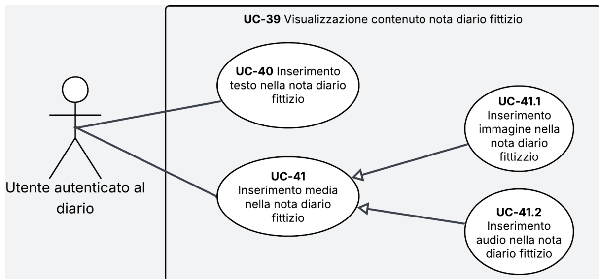
Figura 26: Diagramma dei casi d'uso UC-40, UC-41, UC-41.1 e UC-41.2
