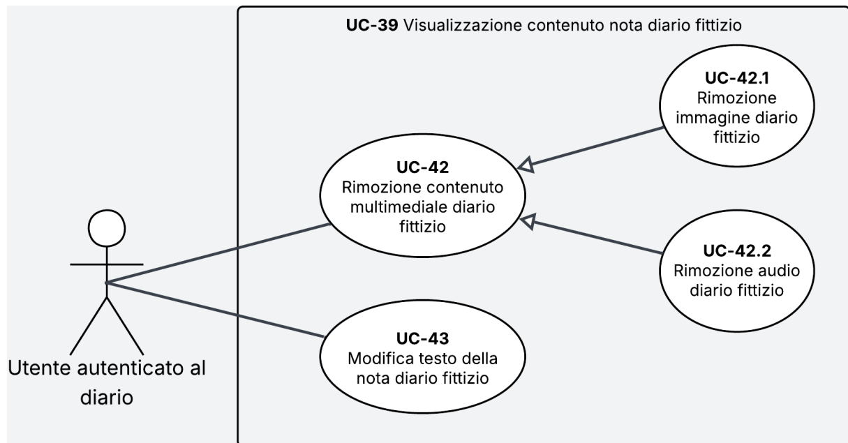
Figura 27: Diagramma dei casi d'uso UC-42, UC-43, UC-42.1 e UC-42.2
