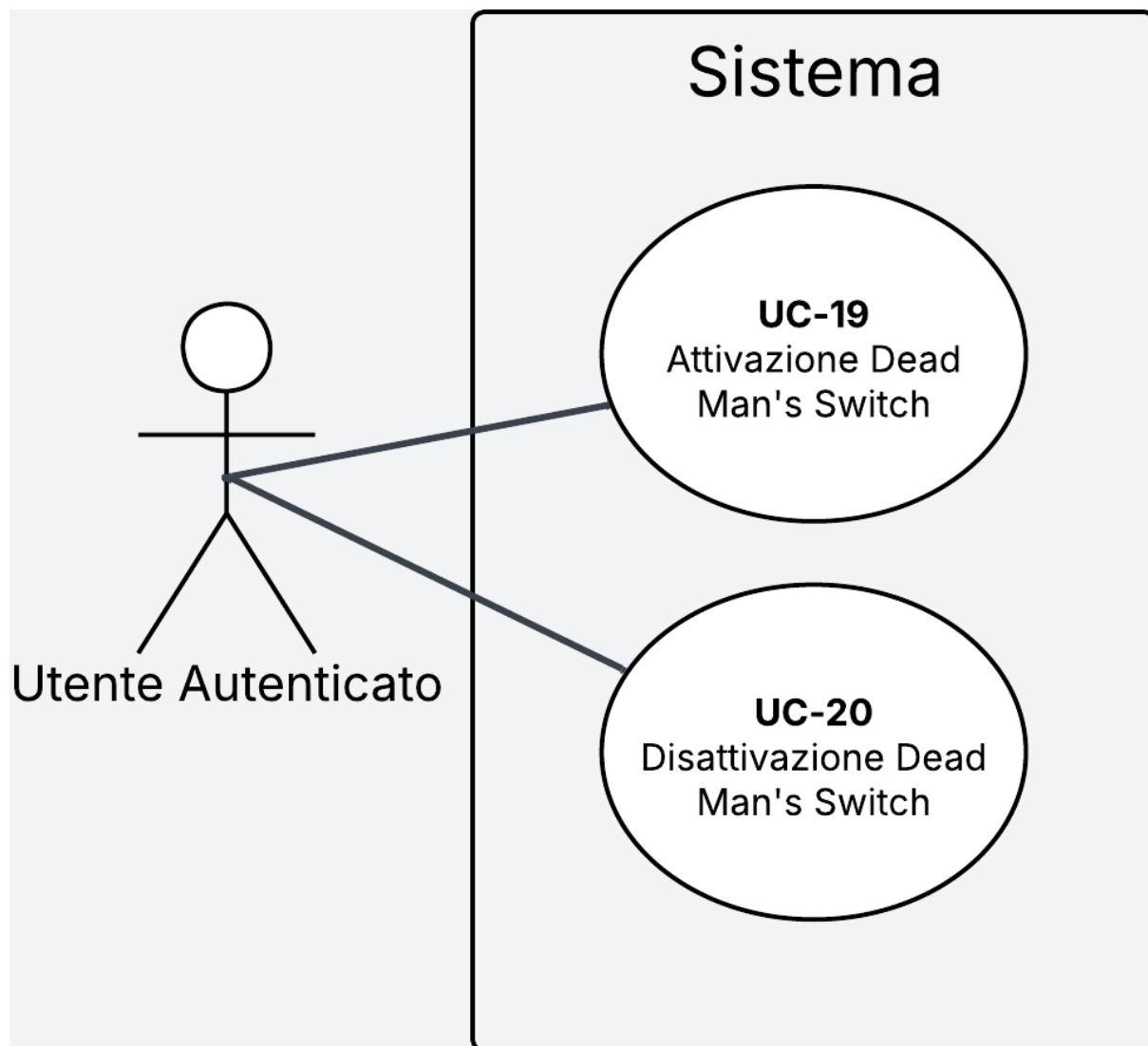
Figura 12: Diagramma dei casi d'uso UC-19 e UC-20
