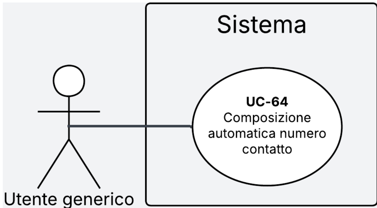
Figura 40: Diagramma del caso d'uso UC-64
