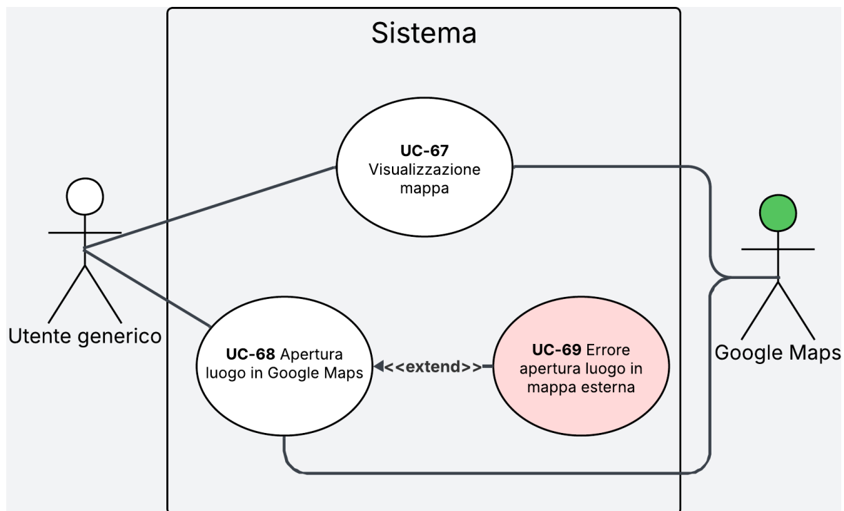
Figura 43: Diagramma del caso d'uso UC-67
