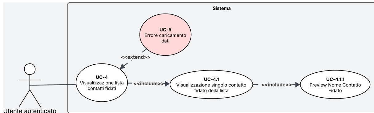
Figura 4: Diagramma del caso d'uso UC-4 con relativi sottocasi d'uso
