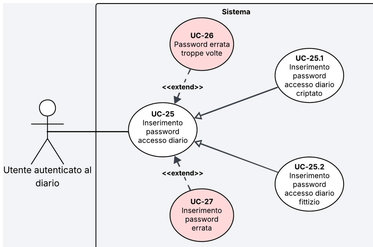
Figura 15: Diagramma del caso d'uso UC-25
