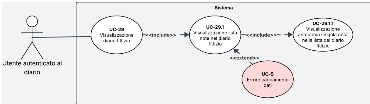
Figura 22: Diagramma del caso d'uso UC-29
