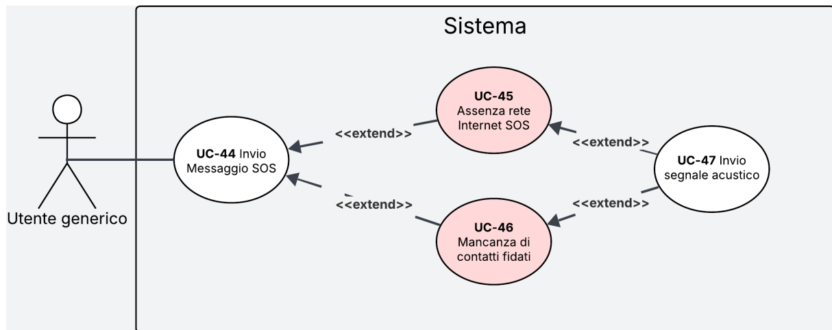
Figura 28: Diagramma del caso d'uso UC-44
