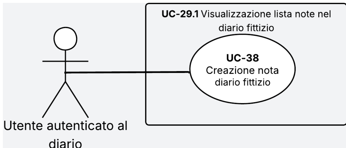
Figura 24: Diagramma del caso d'uso UC-38
