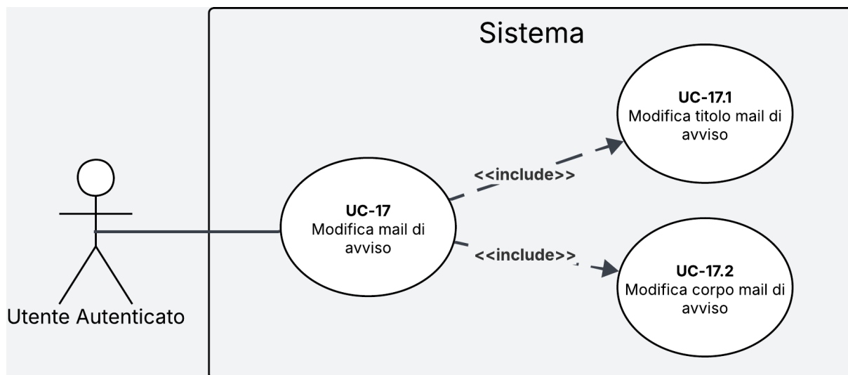
Figura 10: Diagramma del caso d'uso UC-17
