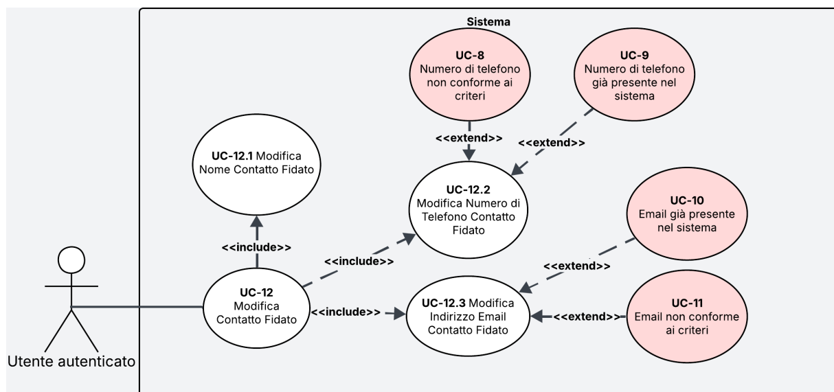
Figura 7: Diagramma del caso d'uso UC-12
