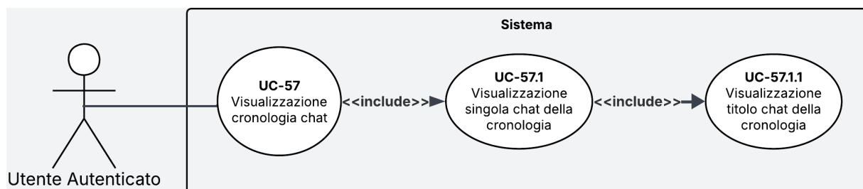
Figura 34: Diagramma del caso d'uso UC-57
