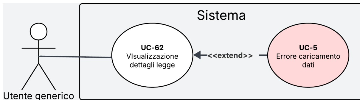
Figura 38: Diagramma del caso d'uso UC-62
