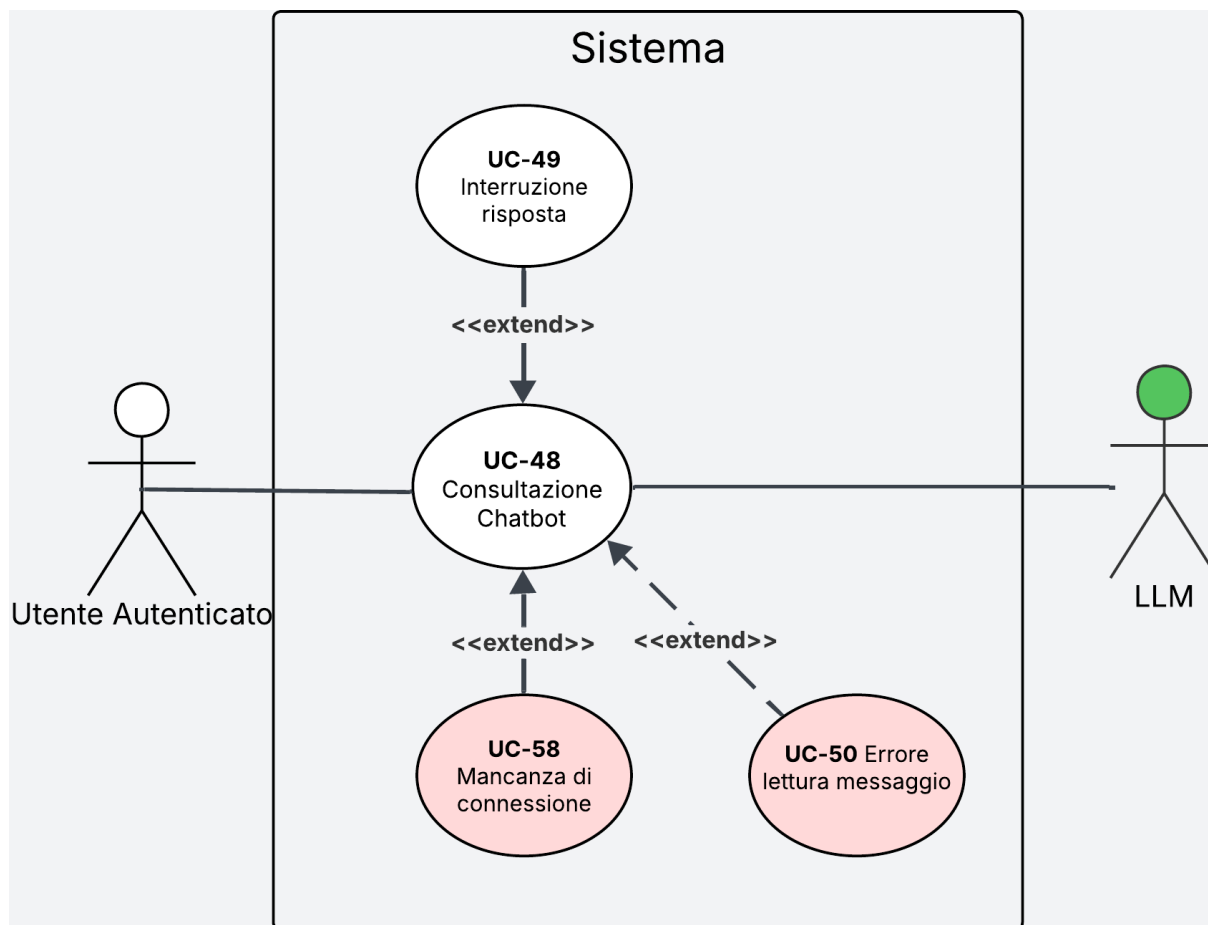
Figura 29: Diagramma del caso d'uso UC-48
