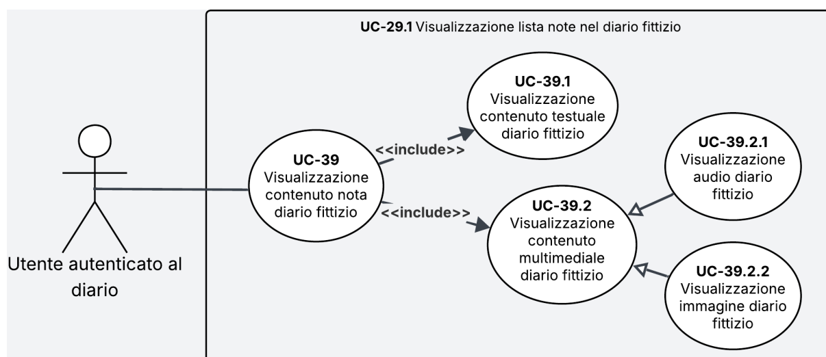
Figura 25: Diagramma del caso d'uso UC-39
