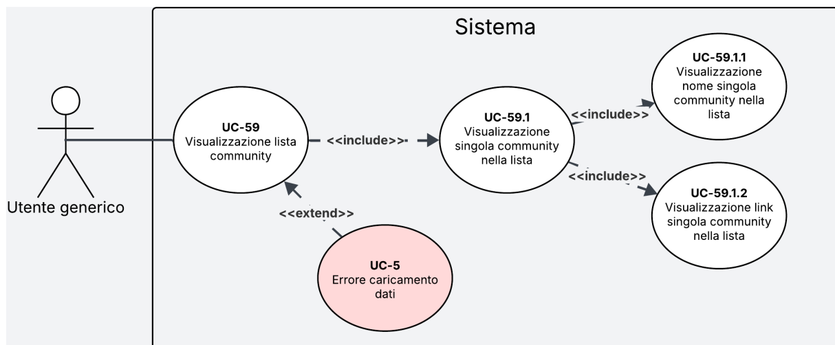
Figura 35: Diagramma del caso d'uso UC-59
