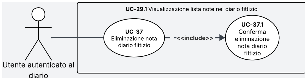
Figura 23: Diagramma dei casi d'uso UC-37 e UC-37.1
