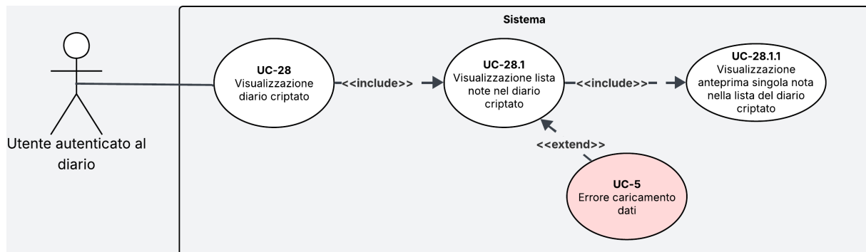
Figura 16: Diagramma del caso d'uso UC-28
