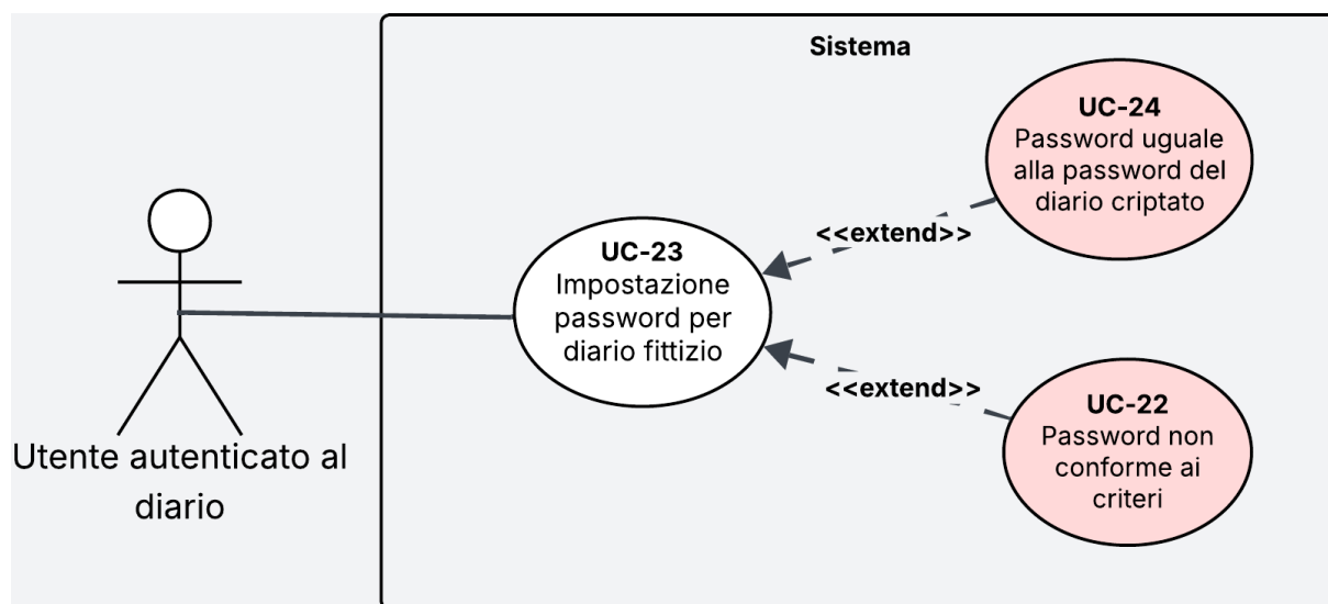
Figura 14: Diagramma del caso d'uso UC-23
