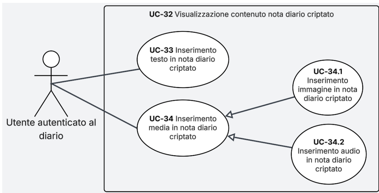
Figura 20: Diagramma dei casi d'uso UC-33, UC-34, UC-34.1 e UC-34.2
