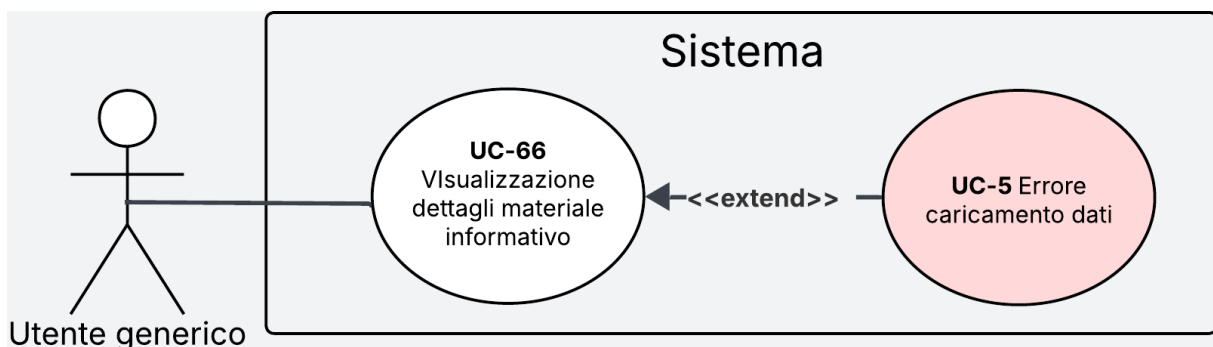
Figura 42: Diagramma del caso d'uso UC-66
