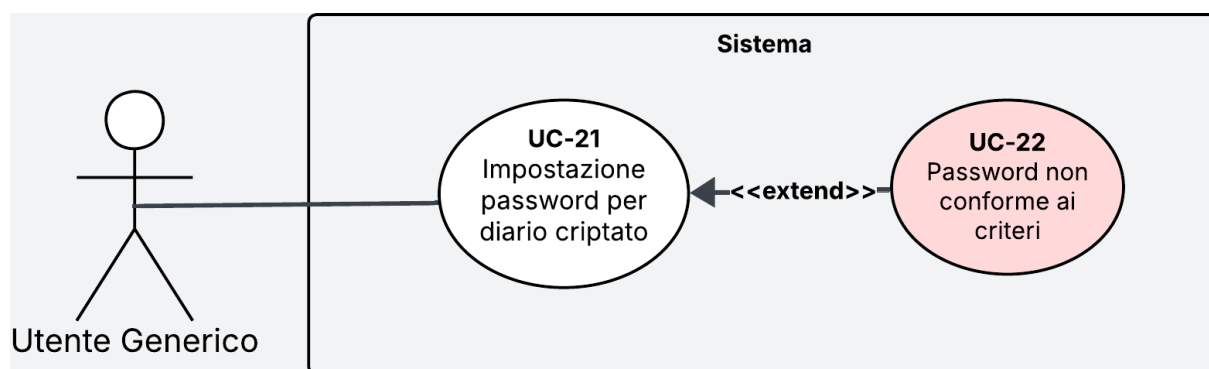
Figura 13: Diagramma del caso d'uso UC-21
