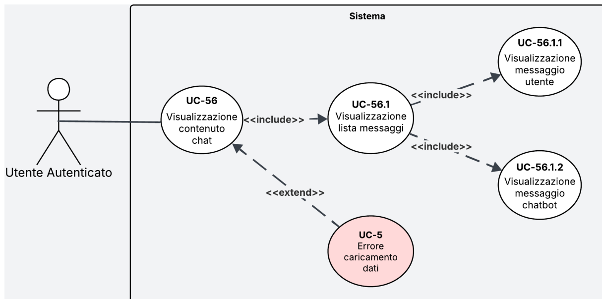
Figura 32: Diagramma del caso d'uso UC-56
