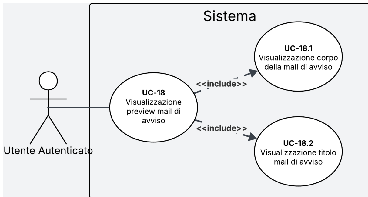
Figura 11: Diagramma del caso d'uso UC-18
