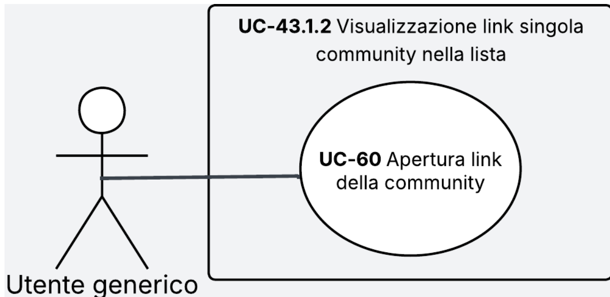
Figura 36: Diagramma del caso d'uso UC-60
