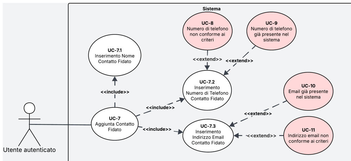
Figura 6: Diagramma del caso d'uso UC-7 con relativi sottocasi d'uso
