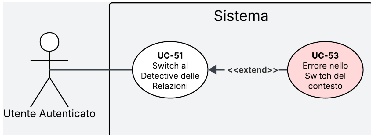
Figura 30: Diagramma del caso d'uso UC-51
