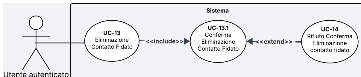
Figura 8: Diagramma del caso d'uso UC-13
