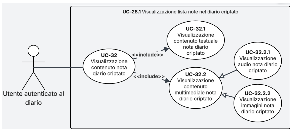
Figura 19: Diagramma del caso d'uso UC-32
