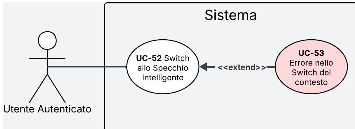
Figura 31: Diagramma del caso d'uso UC-52
