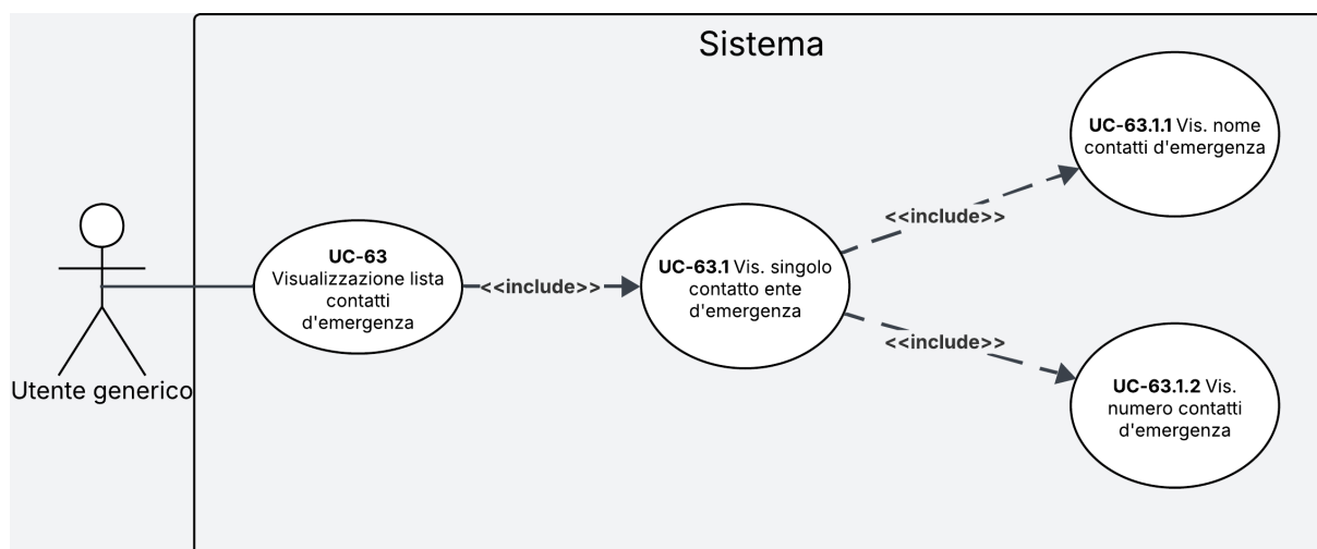
Figura 39: Diagramma del caso d'uso UC-63
