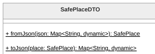
Figura 78: Diagramma della classe SafePlaceDT0
