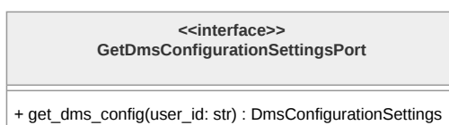
Figura 213: Diagramma della classe GetDmsConfigurationSettingsPort
