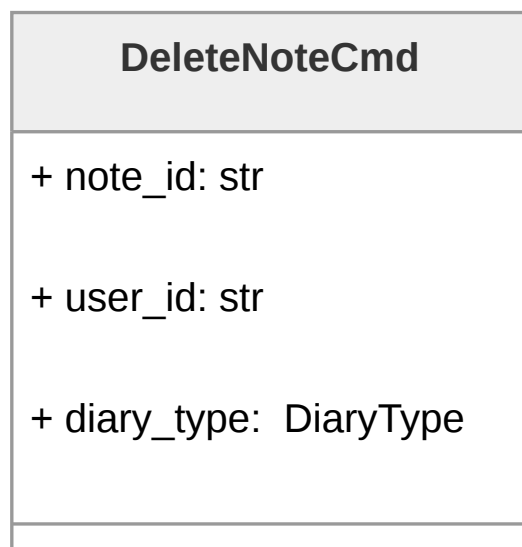
Figura 150: Diagramma della classe DeleteNoteCmd
