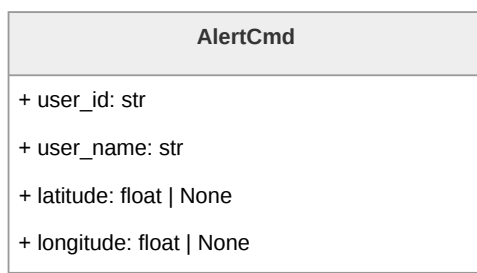
Figura 209: Diagramma della classe AlertCmd
