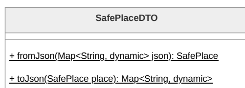
Figura 76: Diagramma della classe SafePlaceDTO
