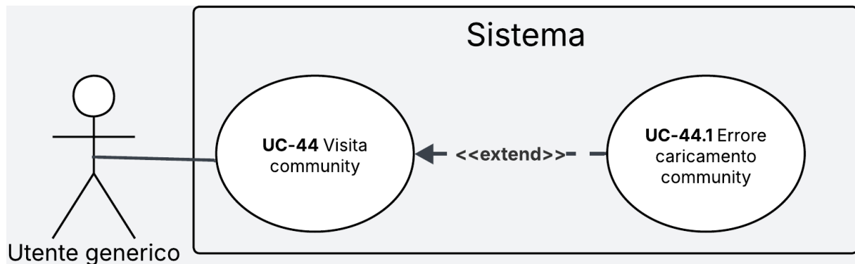
Figura 32: Diagramma del caso d'uso UC-44
