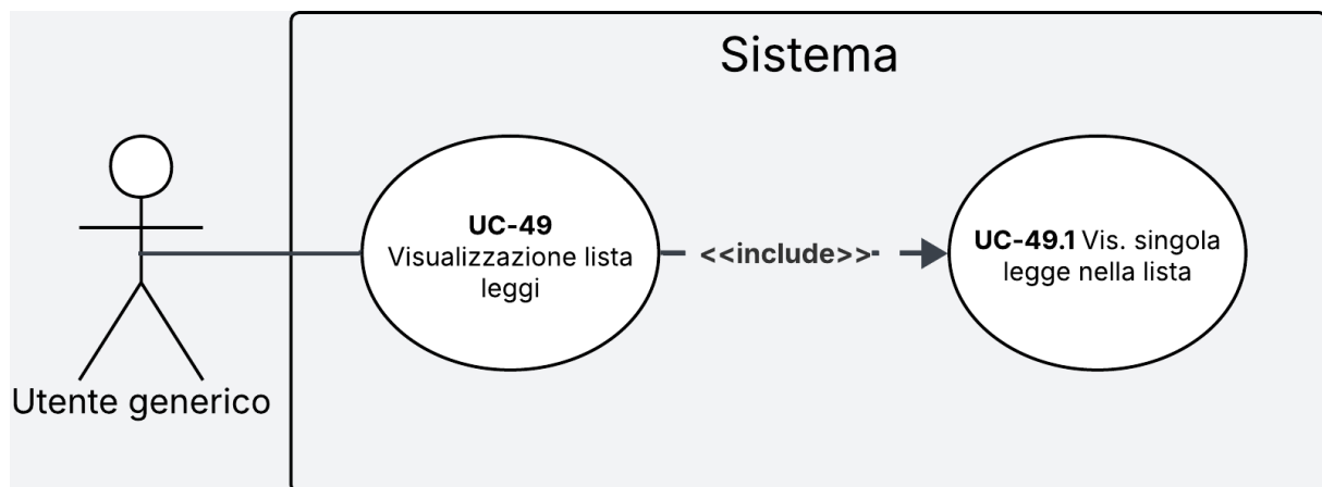
Figura 35: Diagramma del caso d'uso UC-49
