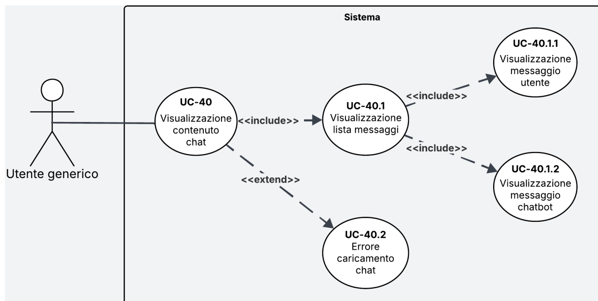
Figura 29: Diagramma del caso d'uso UC-40
