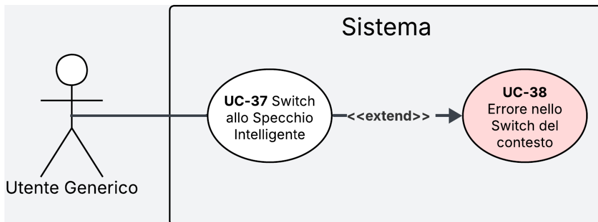
Figura 27: Diagramma del caso d'uso UC-37
