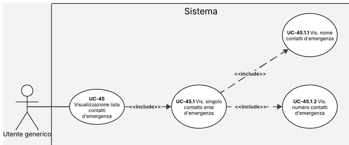
Figura 33: Diagramma del caso d'uso UC-45
