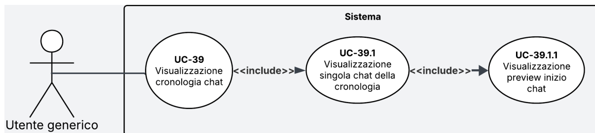
Figura 28: Diagramma del caso d'uso UC-39
