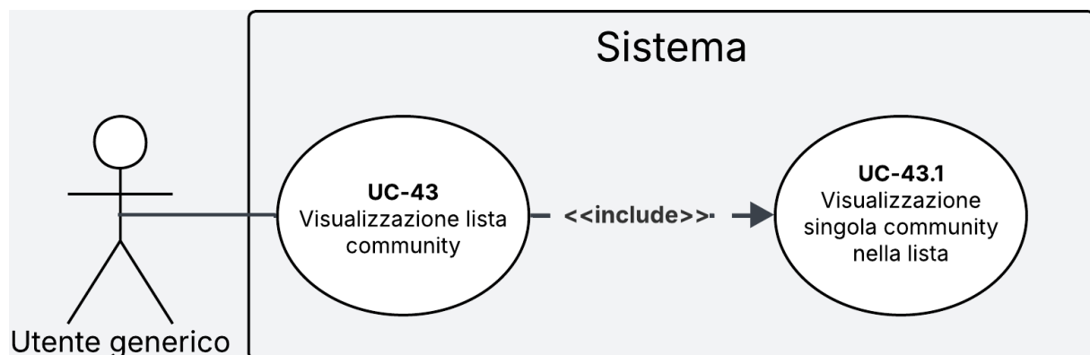
Figura 31: Diagramma del caso d'uso UC-43
