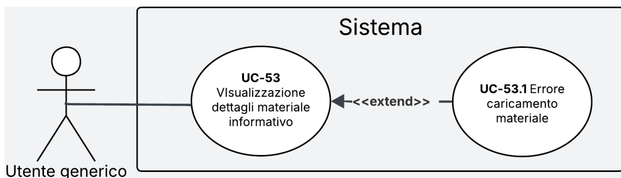
Figura 38: Diagramma del caso d'uso UC-53
