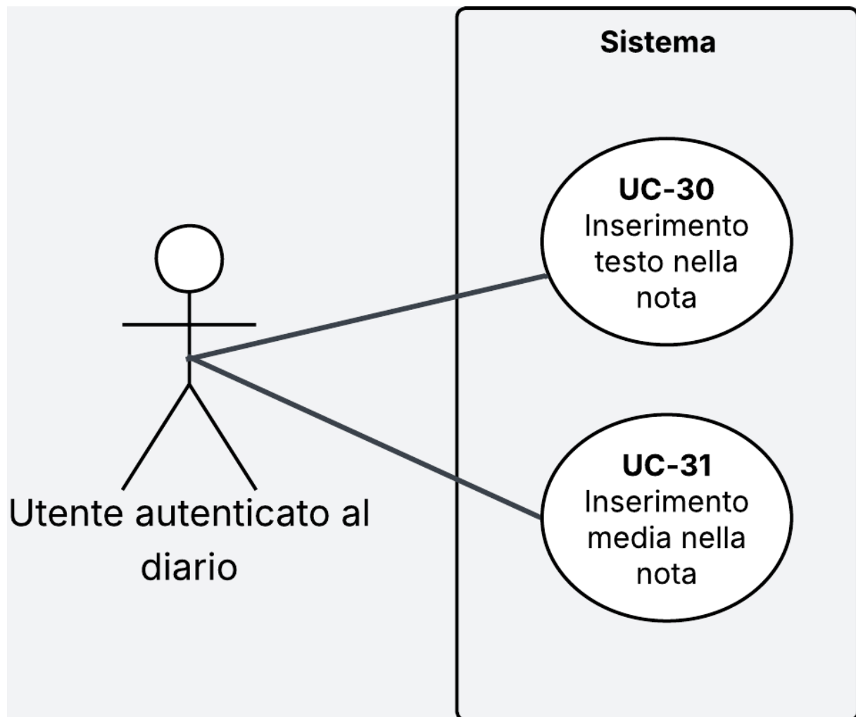
Figura 22: Diagramma dei casi d'uso UC-30 e UC-31
