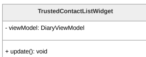
Figura 61: Diagramma della classe TrustedContactListWidget
