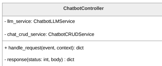
Figura 180: Diagramma della classe ChatBotController
