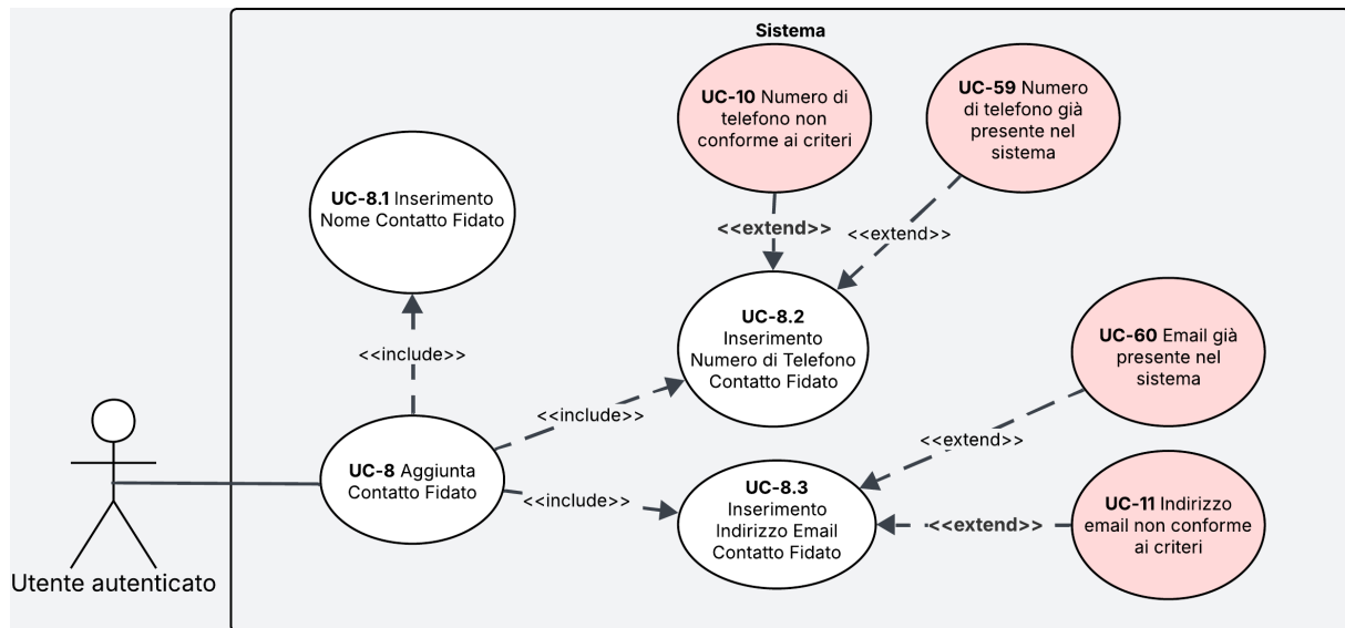
Figura 6: Diagramma del caso d'uso UC-8
