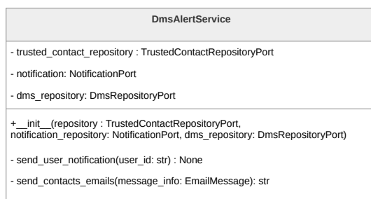
Figura 184: Diagramma della classe DmsAlertService
