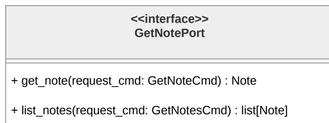
Figura 157: Diagramma dell'interfaccia GetNotePort
