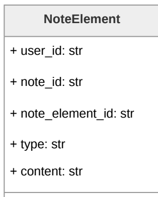
Figura 145: Diagramma della classe NoteElement
