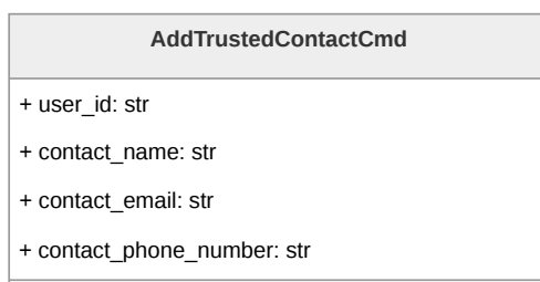
Figura 205: Diagramma della classe AddTrustedContactCmd
