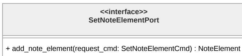
Figura 160: Diagramma dell'interfaccia SetNoteElementPort
