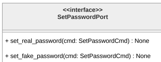
Figura 144: Diagramma dell'interfaccia SetPasswordPort
