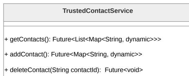
Figura 9: Diagramma della classe TrustedContactService
