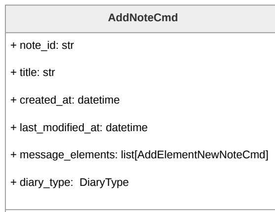
Figura 149: Diagramma della classe AddNoteCmd
