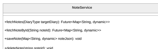
Figura 64: Diagramma della classe NoteService
