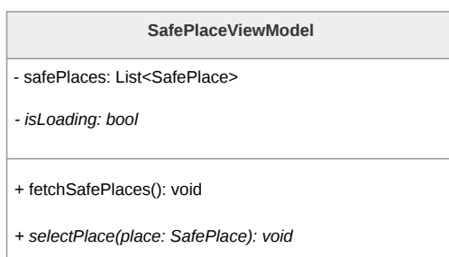
Figura 80: Diagramma della classe SafePlaceViewModel
