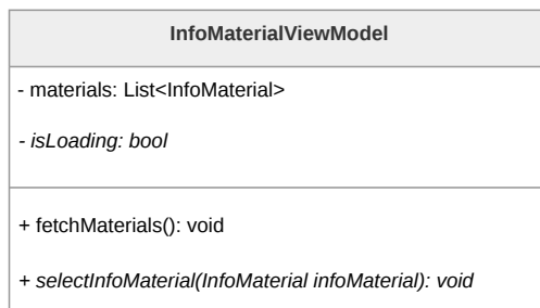
Figura 111: Diagramma della classe InfoMaterialViewModel
