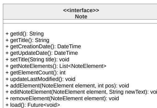
Figura 57: Diagramma della classe Note
