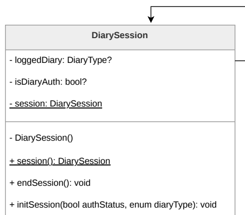
Figura 55: Diagramma della classe DiarySession
