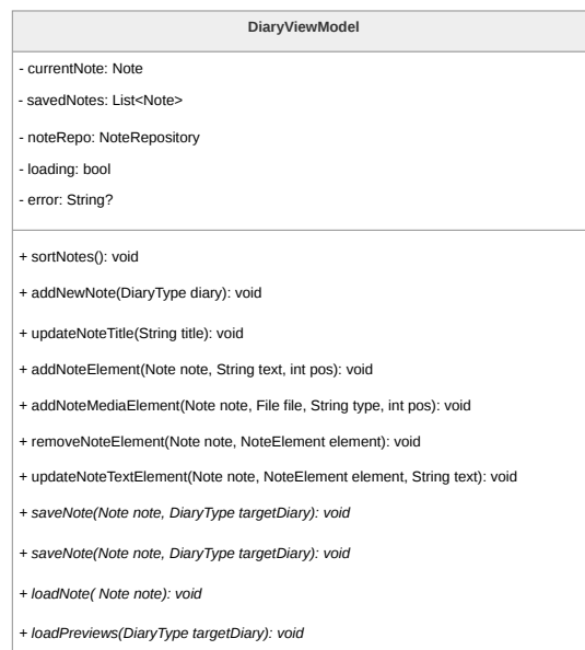
Figura 54: Diagramma della classe DiaryViewModel
