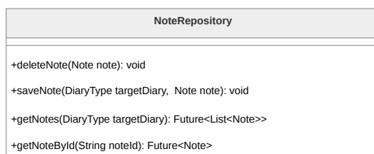
Figura 65: Diagramma della classe NoteRepository
