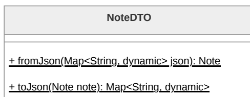
Figura 66: Diagramma della classe NoteDTO
