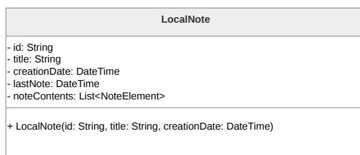
Figura 59: Diagramma della classe LocalNote
