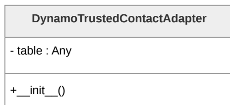
Figura 189: Diagramma della classe DynamoTrustedContactAdapter
