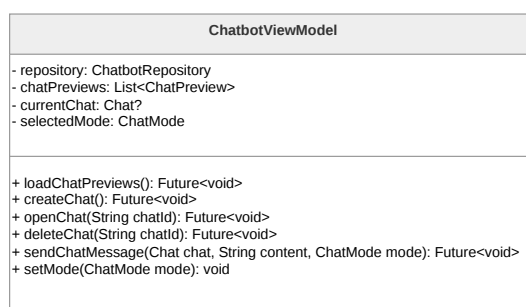
Figura 8: Diagramma della classe ChatbotViewModel
