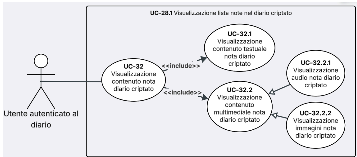
Figura 20: Diagramma del caso d'uso UC-32
