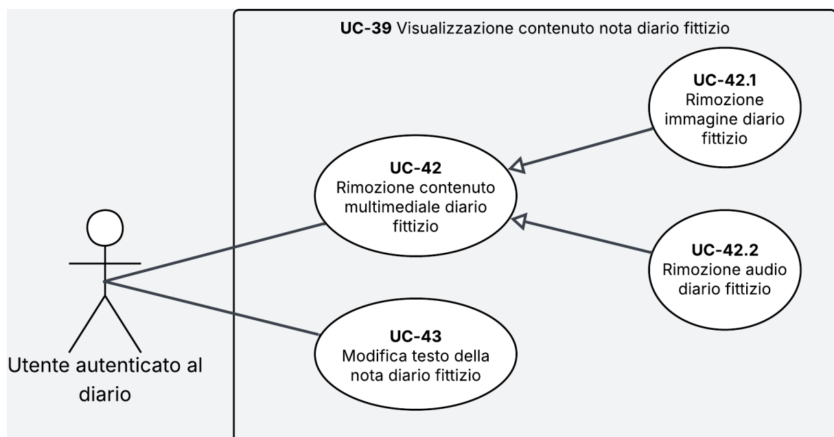
Figura 21: Diagramma dei casi d'uso UC-42, UC-43, UC-42.1 e UC-42.2
