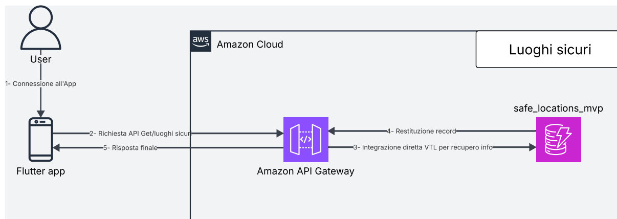
Figura 116: Architettura G moduli Luoghi Sicuri
