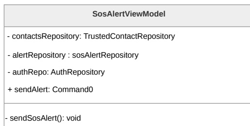
Figura 12: Diagramma delle classe SosAlertViewModel
