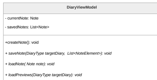
Figura 46: Diagramma della classe DiaryViewModel
