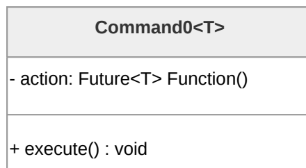
Figura 16: Diagramma delle classe Command0<T>
