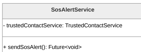
Figura 14: Diagramma delle classe SosAlertService
