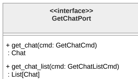
Figura 152: Diagramma dell'interfaccia GetChatPort
