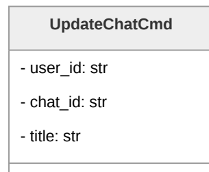
Figura 160: Diagramma della classe UpdateChatCmd
