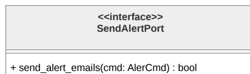
Figura 185: Diagramma della classe SendAlertPort
