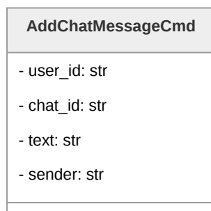
Figura 162: Diagramma della classe AddChatMessageCmd
