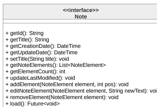
Figura 58: Diagramma della classe Note
