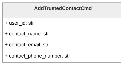
Figura 170: Diagramma della classe AddTrustedContactCmd
