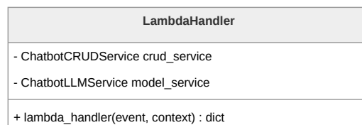
Figura 165: Diagramma della classe LambdaHandler
