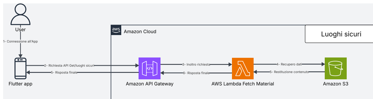
Figura 125: Architettura moduli Luoghi Sicuri
