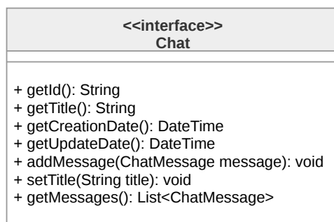
Figura 144: Diagramma della classe Chat
