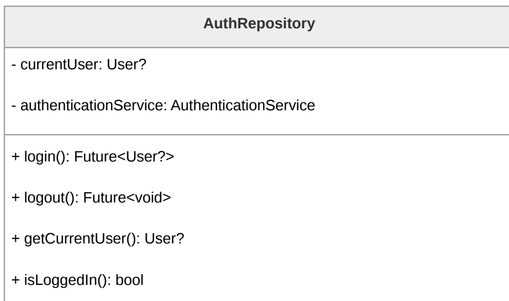
Figura 17: Diagramma della classe AuthRepository
