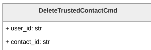
Figura 207: Diagramma della classe DeleteTrustedContactCmd
