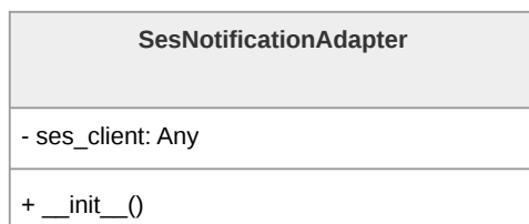
Figura 230: Diagramma della classe SesNotificationAdapter
