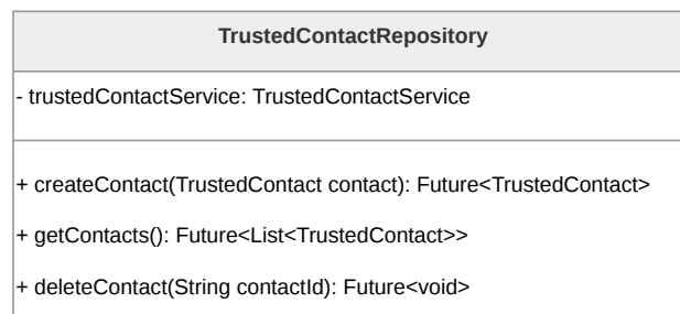
Figura 75: Diagramma della classe TrustedContactRepository
