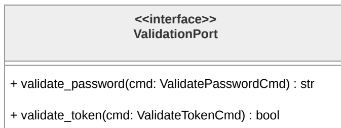
Figura 163: Diagramma dell'interfaccia ValidationPort
