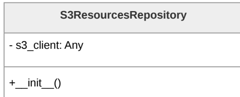
Figura 140: Diagramma della classe S3ResourcesRepository
