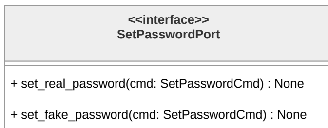
Figura 162: Diagramma dell'interfaccia SetPasswordPort
