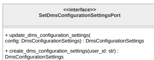
Figura 215: Diagramma della classe SetDmsConfigurationSettingsPort
