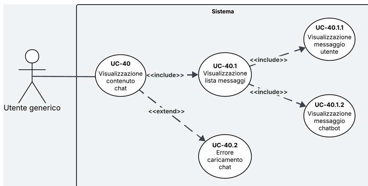
Figura 33: Diagramma del caso d'uso UC-40
