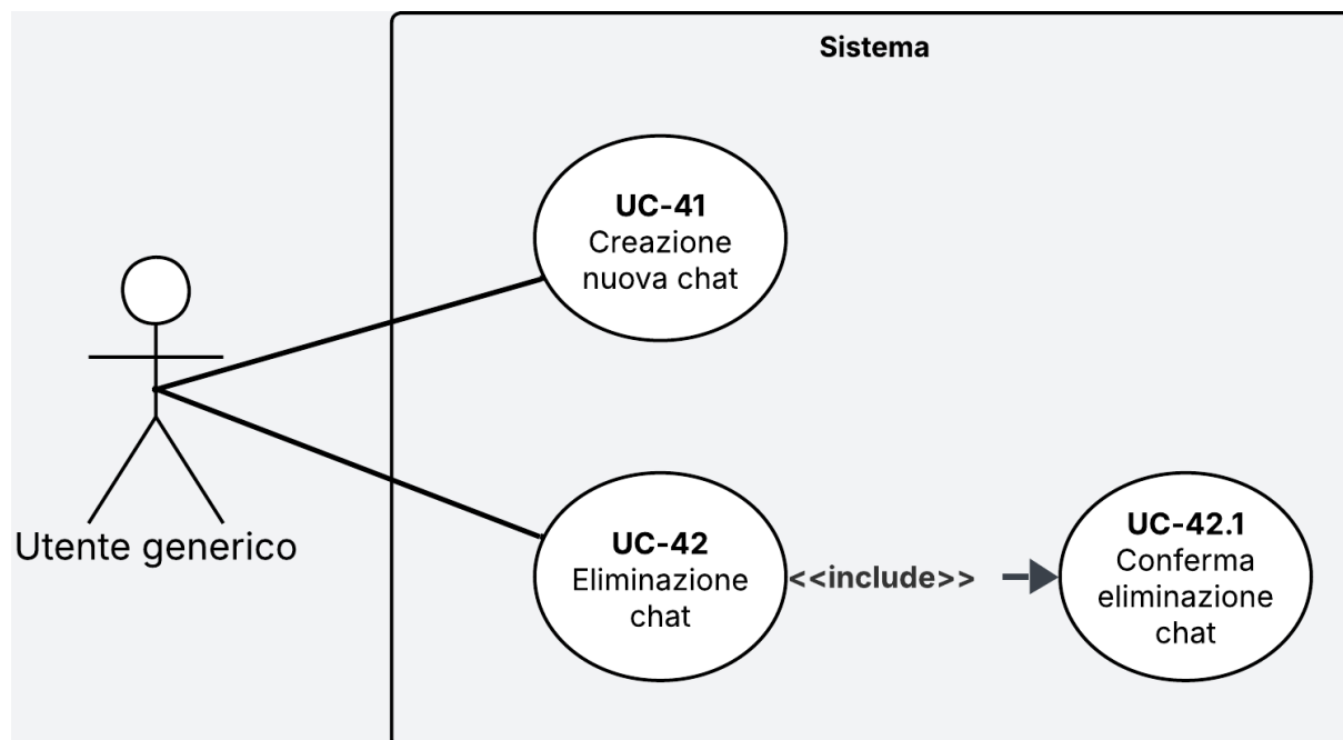
Figura 34: Diagramma dei casi d'uso UC-41 e UC-42
