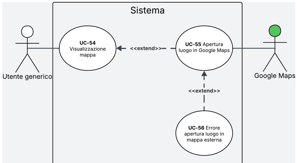
Figura 43: Diagramma del caso d'uso UC-54
