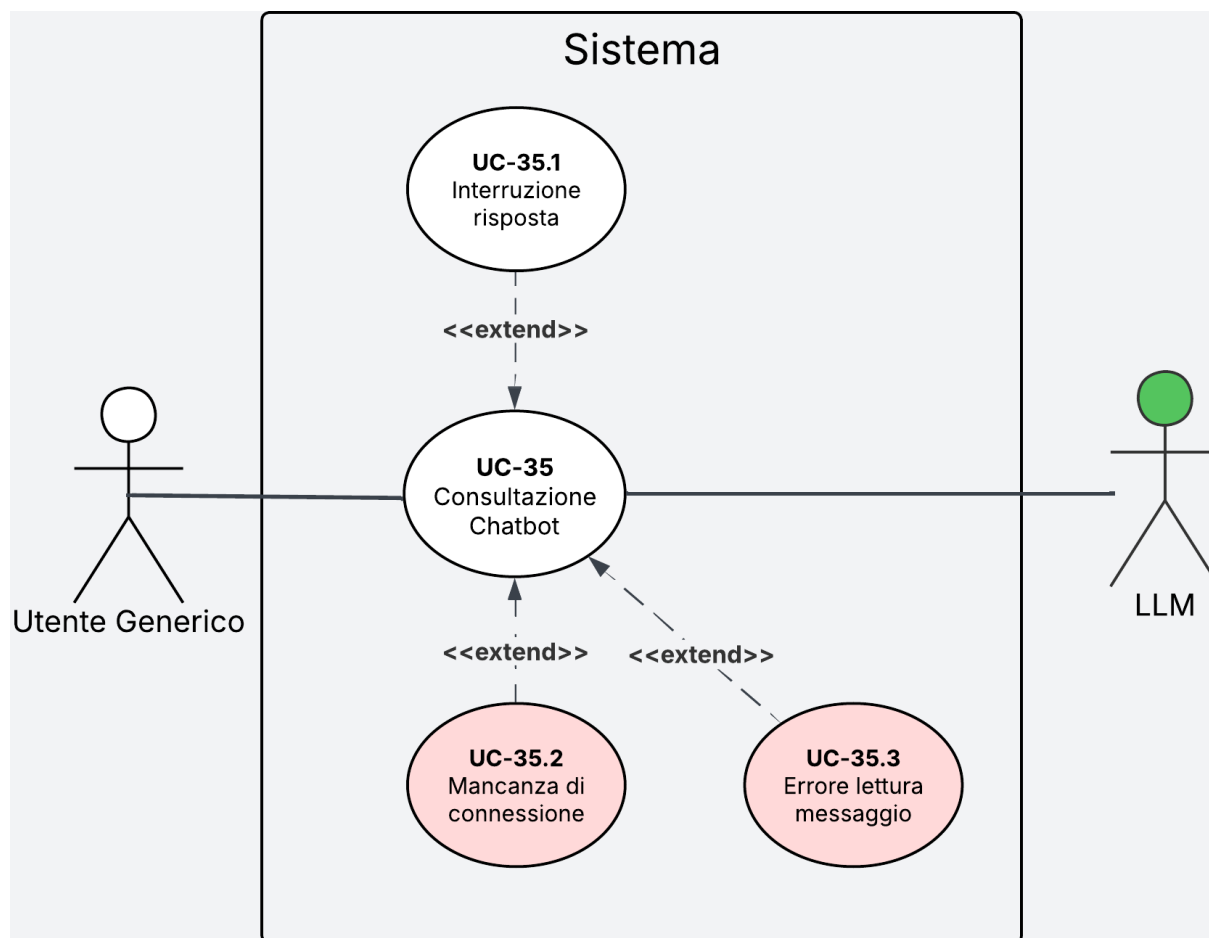
Figura 29: Diagramma del caso d'uso UC-35
