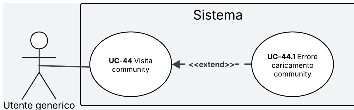
Figura 36: Diagramma del caso d'uso UC-44
