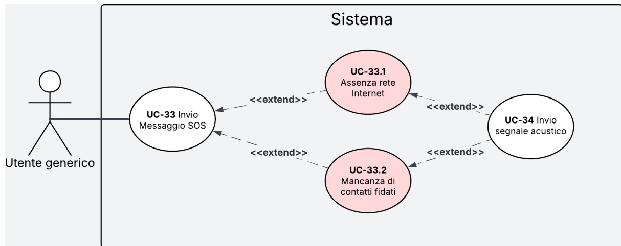
Figura 28: Diagramma del caso d'uso UC-33
