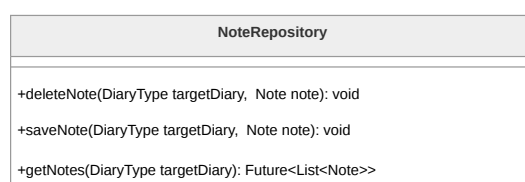
Figura 57: Diagramma della classe NoteRepository
