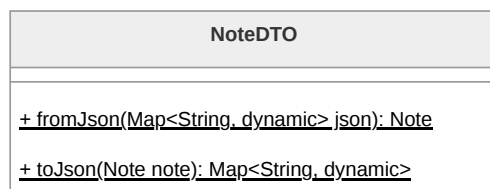
Figura 58: Diagramma della classe NoteDTO
