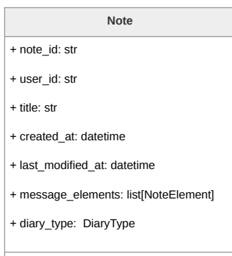
Figura 124: Diagramma della classe Note
