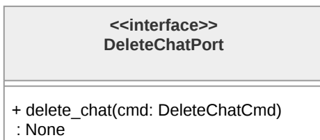
Figura 169: Diagramma dell'interfaccia DeleteChatPort
