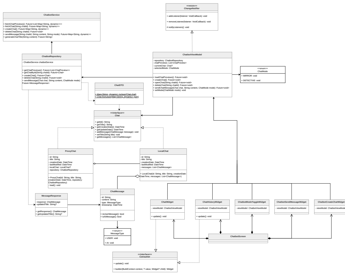
Figura 24: Diagramma delle classi relativo alle funzionalità del Chatbot
