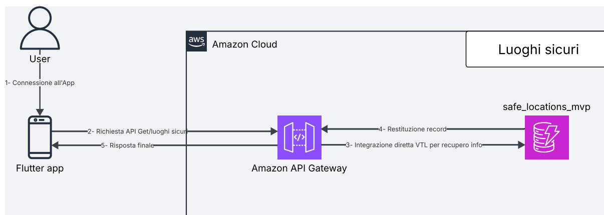
Figura 91: Architettura G moduli Luoghi Sicuri
