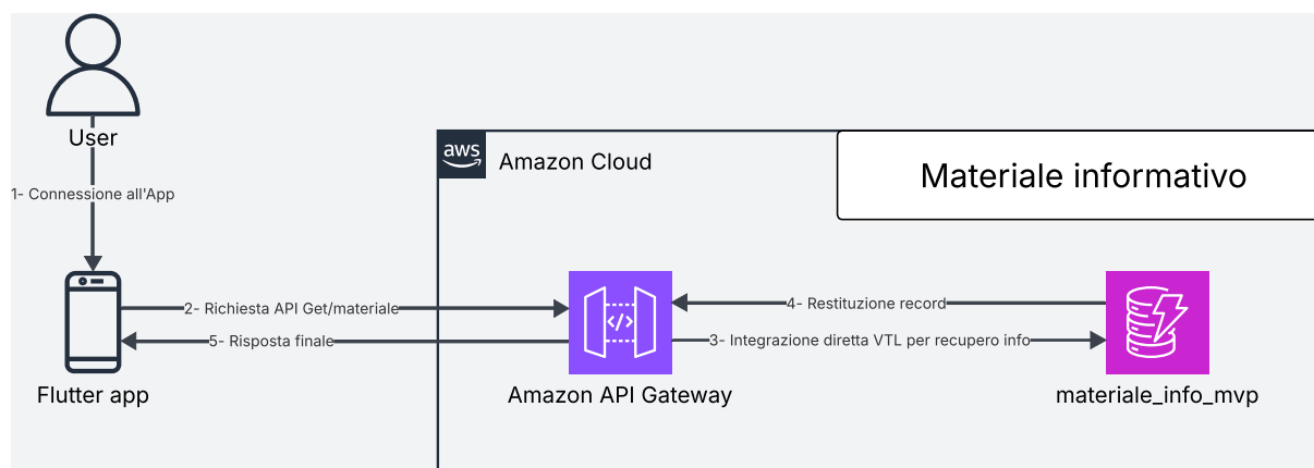
Figura 92: Architettura G moduli Materiale Informativo
