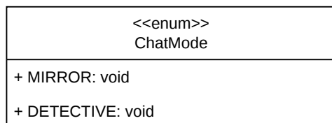
Figura 13: Diagramma della classe ChatMode
