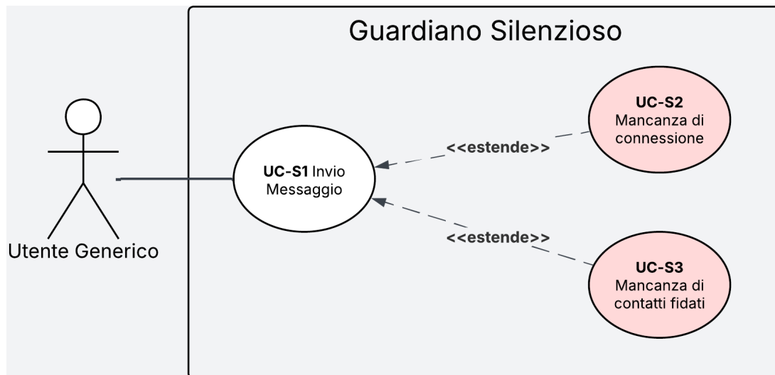
Figura 12: Diagramma del caso d'uso UC-S1 con UC-S2 e UC-S3
