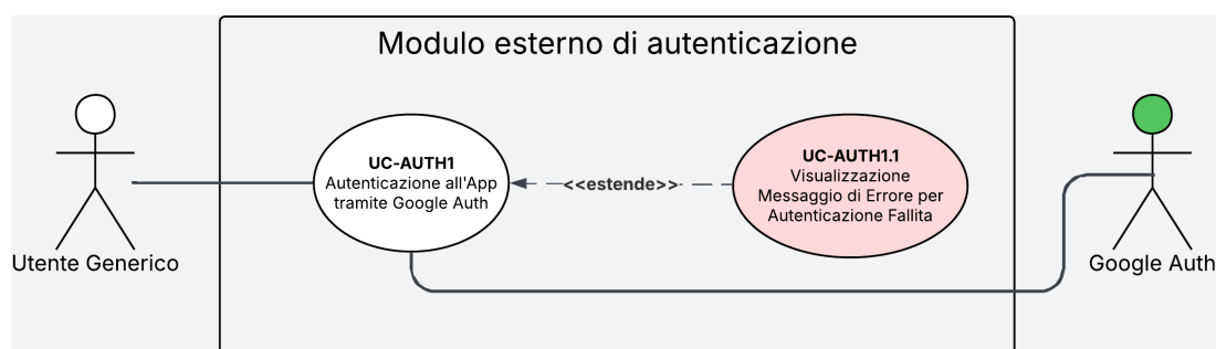
Figura 1: Diagramma dei casi d'uso UC-AUTH1 e UC-AUTH1.1
