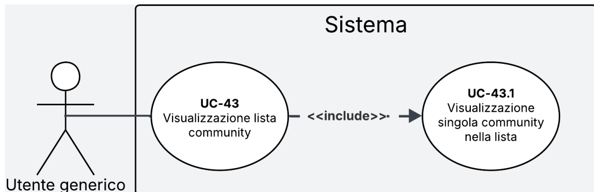
Figura 29: Diagramma del caso d'uso UC-43
