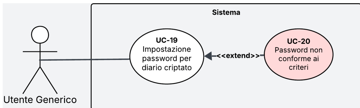
Figura 13: Diagramma del caso d'uso UC-19
