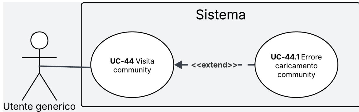
Figura 30: Diagramma del caso d'uso UC-44
