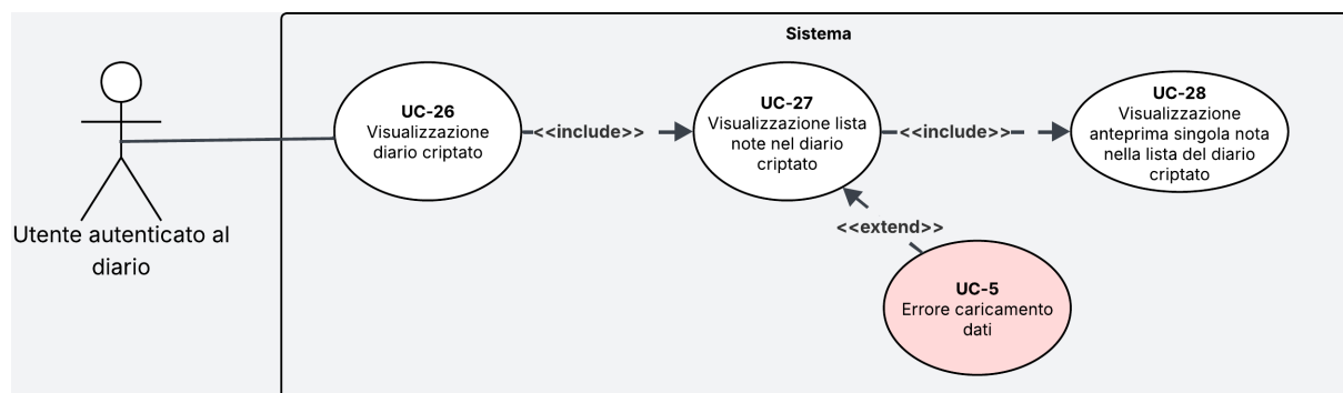
Figura 16: Diagramma del caso d'uso UC-26
