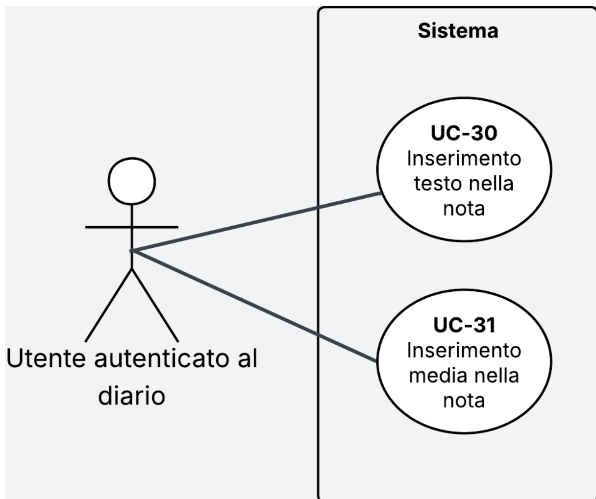
Figura 20: Diagramma dei casi d'uso UC-30 e UC-31
