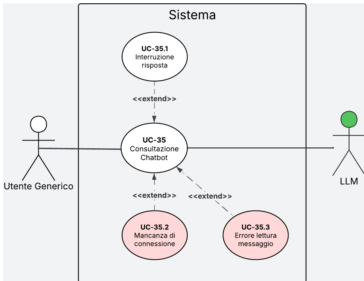
Figura 23: Diagramma del caso d'uso UC-35
