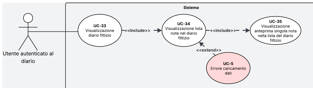
Figura 17: Diagramma del caso d'uso UC-33
