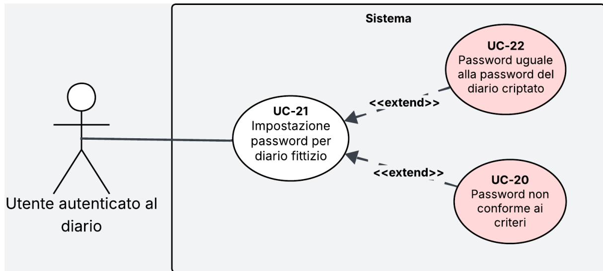
Figura 14: Diagramma del caso d'uso UC-21
