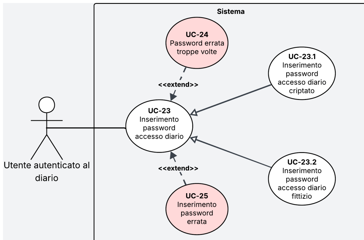
Figura 15: Diagramma del caso d'uso UC-23
