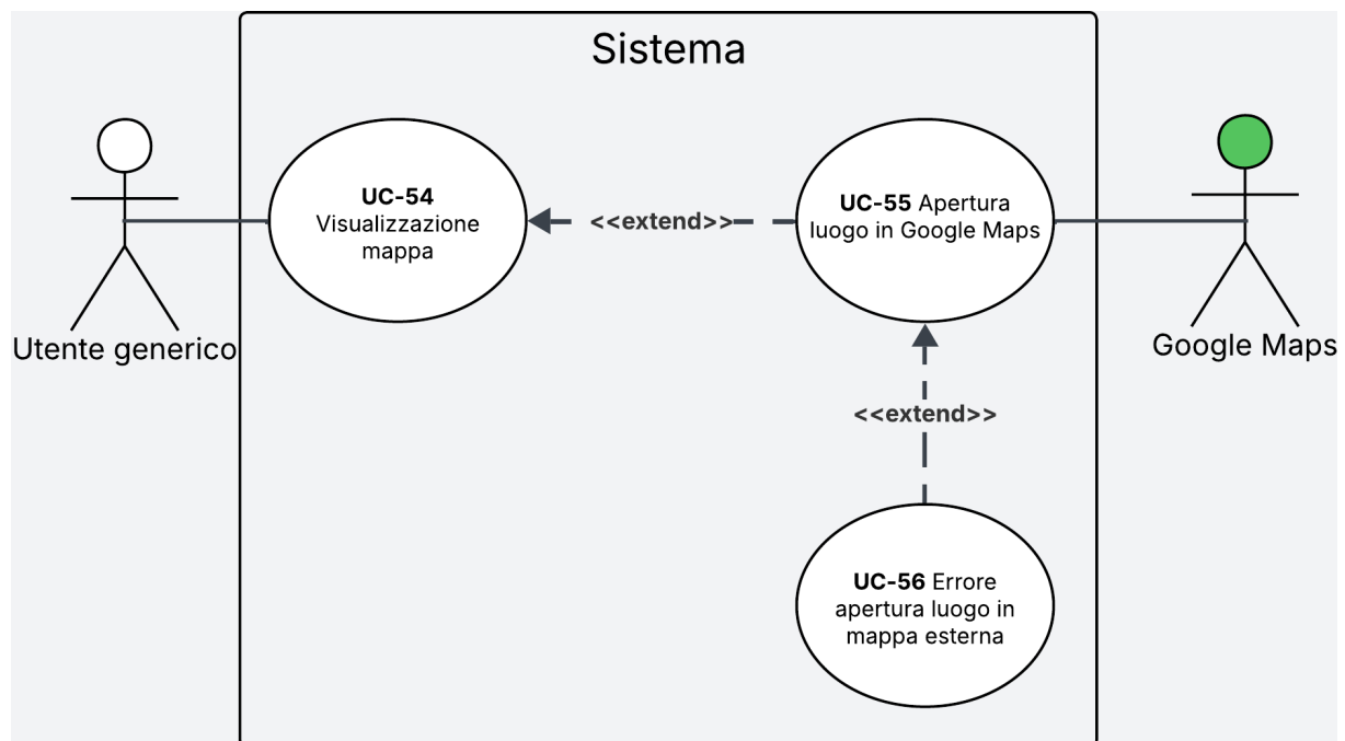
Figura 37: Diagramma del caso d'uso UC-54
