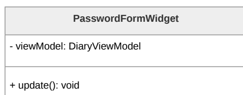
Figura 21: Diagramma della classe PasswordFormWidget
