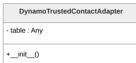
Figura 191: Diagramma della classe DynamoTrustedContactAdapter
